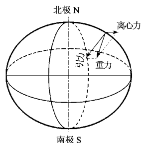
图 1-1 地球重力
