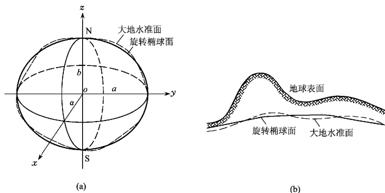
图 1-3 旋转椭球 (a)整体略图;(b)局部示意图
