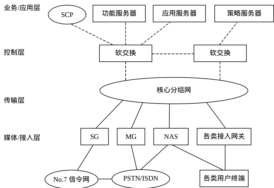
图 1-2 软交换系统结构示意图
