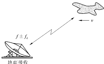
图 1-1-2 多普勒效应
