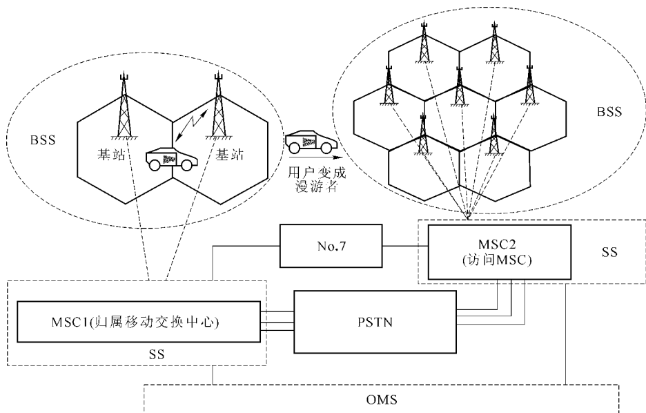
图 1-1 移动通信系统的组成
