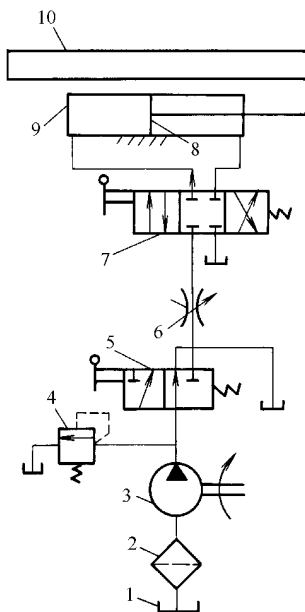
图 1-10 用图形符号表示的磨床液压系统
