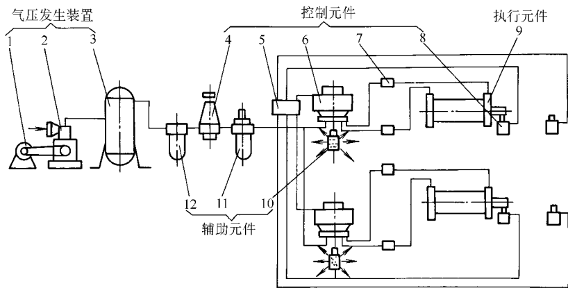
图 1-1-1 气动系统的组成示意图
