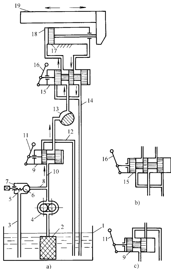
图 1-1 磨床工作台液压系统工作原理图
