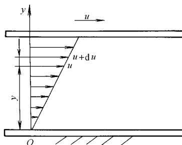
图 2-1 液体粘性示意图
