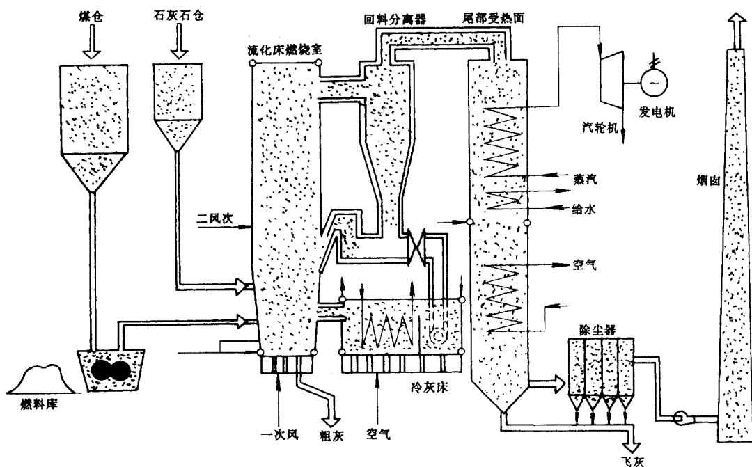
图 1-3 带外置换热器的循环流化床锅炉流程
