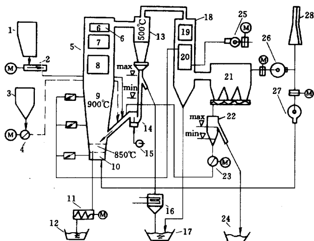
图 1-4 Circofluid 型循环流化床锅炉工艺流程
