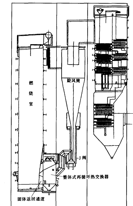
图 1-2 CFB 锅炉
