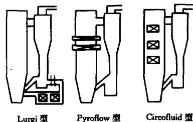
图 1-1 各种循环流化床燃烧装置
