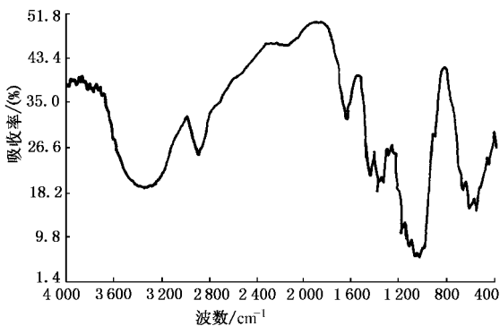
图圆-员 棕色棉的红外吸收光谱图
