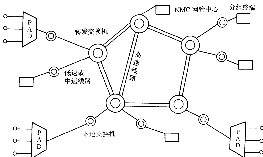
图 1.15 分组交换网的基本结构
