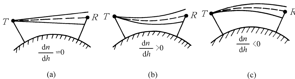
图 1.11 电波折射的波束轨迹
