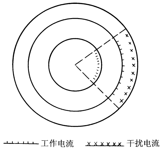
图 1.7 同轴回路中的工作电流和干扰电流
