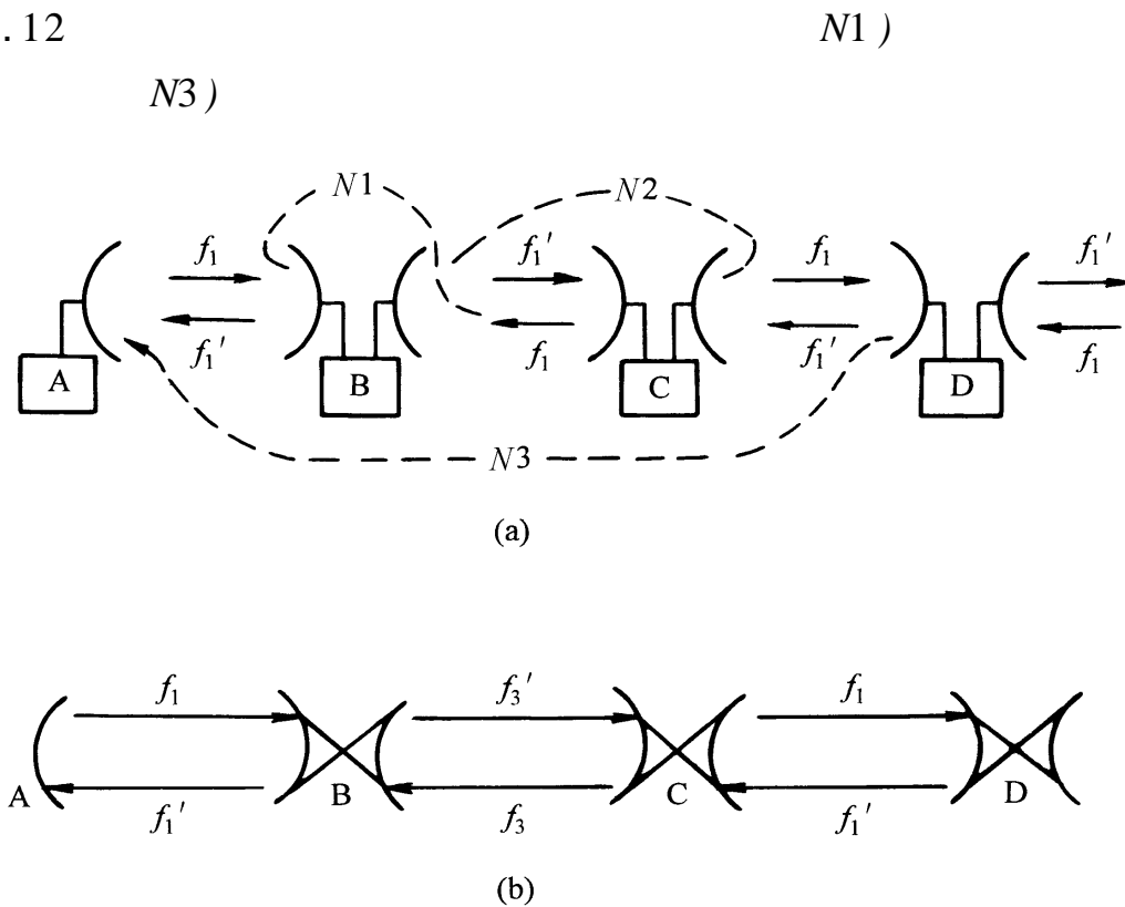
图 1.12 双向传输频率配置
