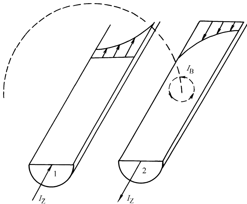
图 1.3 靠近效应示意图
