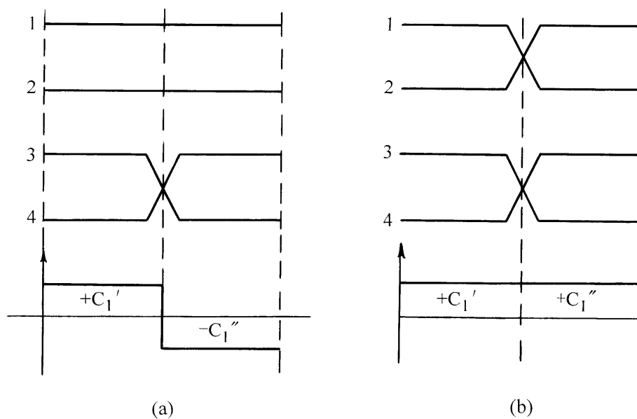
图 1.8 交叉的作用示意图
