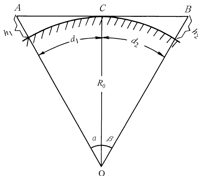
图 1.10 地球曲率对视距的影响
