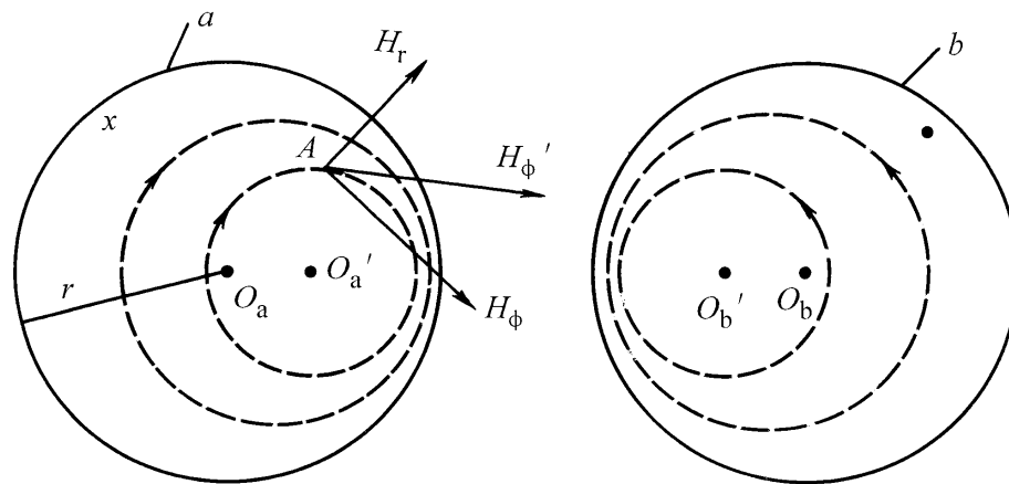
图 1.5 对称回路导线截面上磁场分布图
