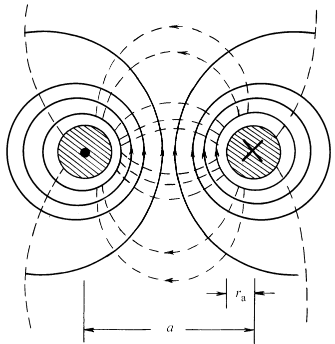
图 1.4 对称回路导线间电磁场分布
