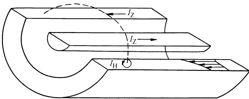
图 1.6 同轴回路的靠近效应
