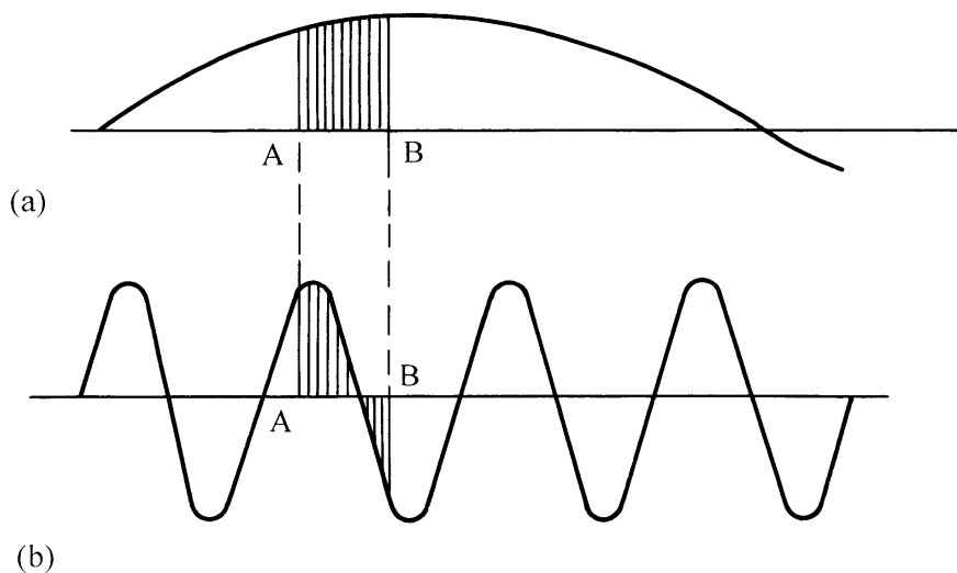
图 1.2 正弦电压沿线相位变化示意图
