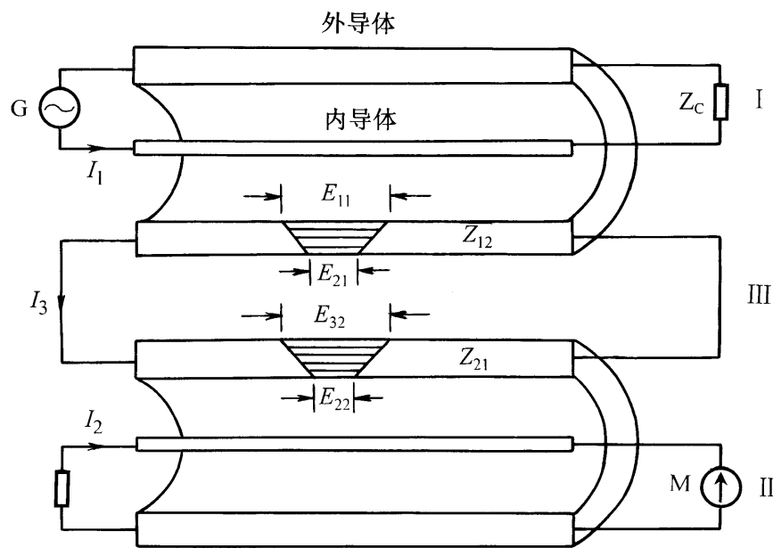
图 1.9 同轴回路间的干扰
