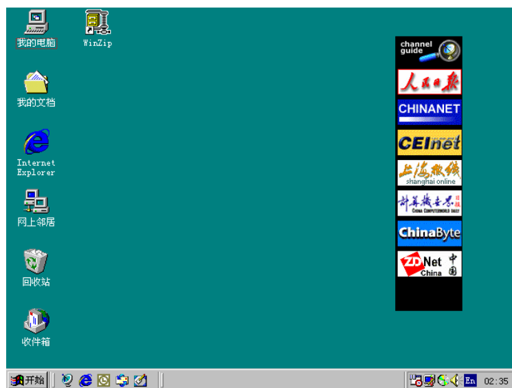
图 1.1 Windows 98 桌面
