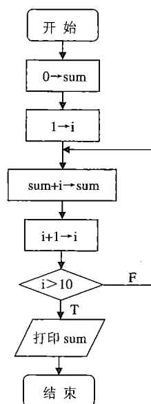
图 1.4 求 \sum_{i=1}^{10} i 算法的程序流程图
