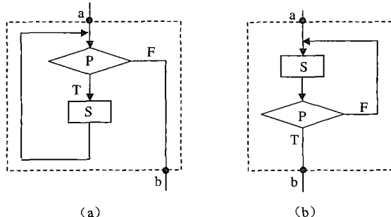
图 1.3 循环结构
