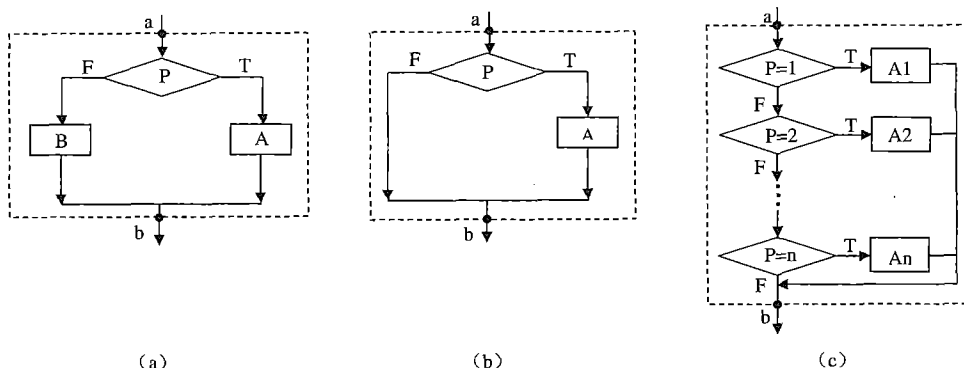
图 1.2 选择结构
