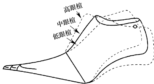
图1-7 不同跟高跟鞋植
