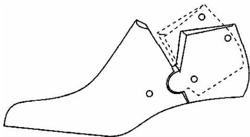
图 1-4 V 字型鞋楦
