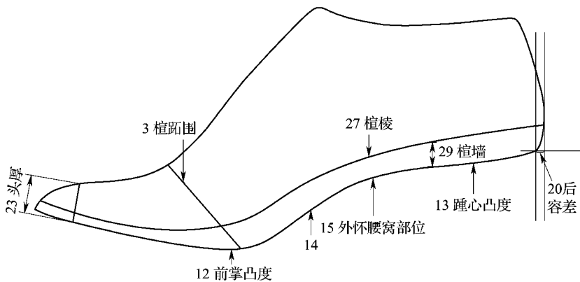
图 1-1 鞋楦各部位名称
