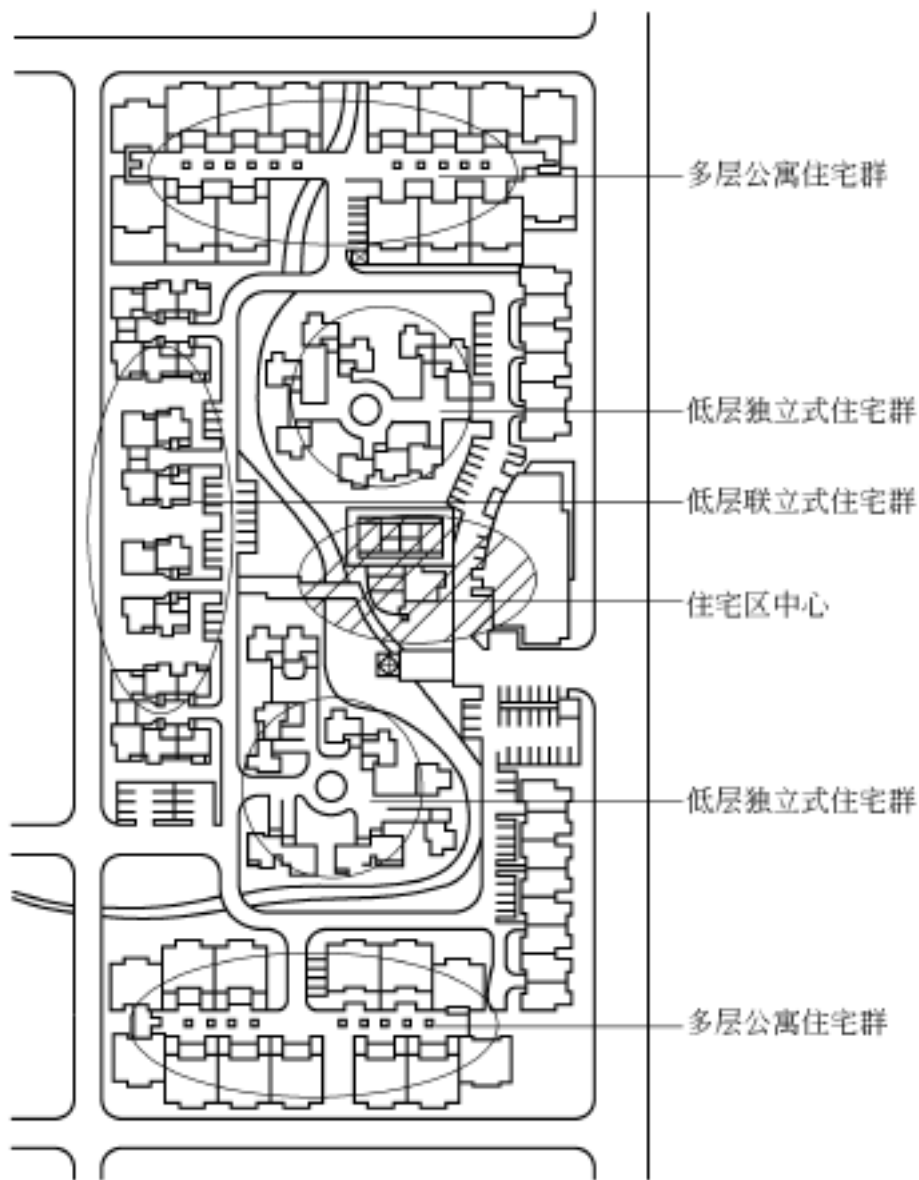
图 1-7 成组成团的组合方式
