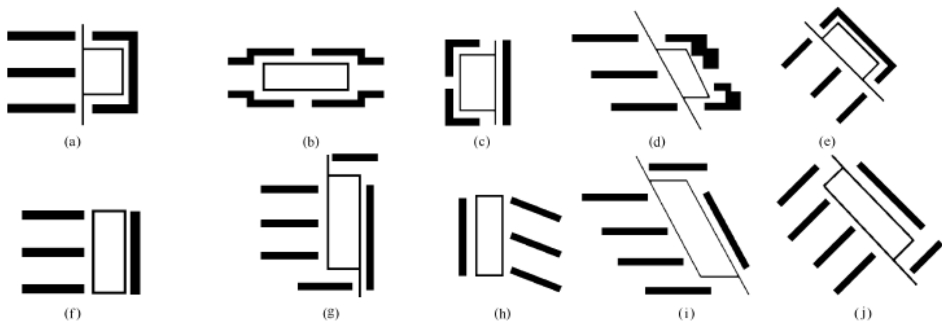
图 1-6c 混合式布置的几种形式
