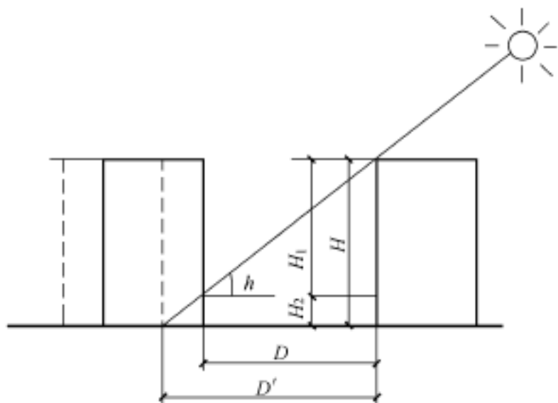
图 1-1 平地日照间距计算图
