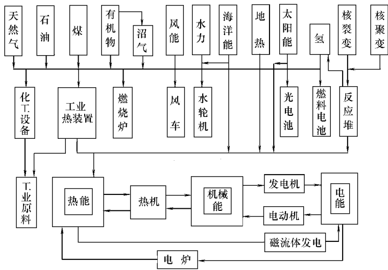
图 圆 主要能源及其转化和应用
