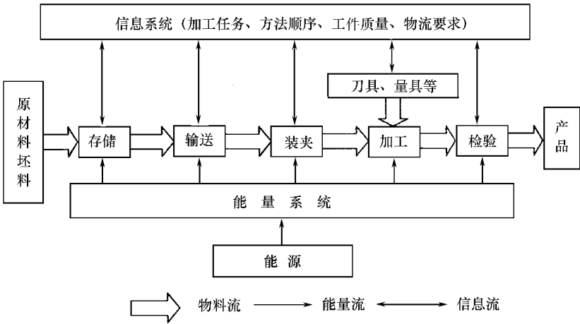
图 园源 机械制造系统组成图
