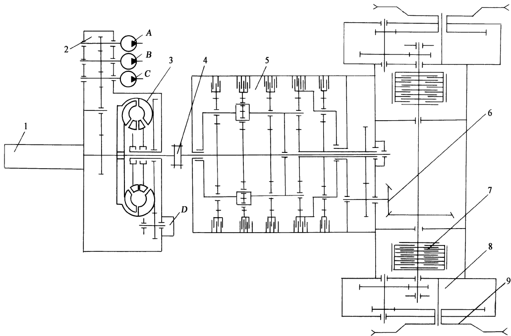
图 远 推土机液力机械式传动系布置简图
