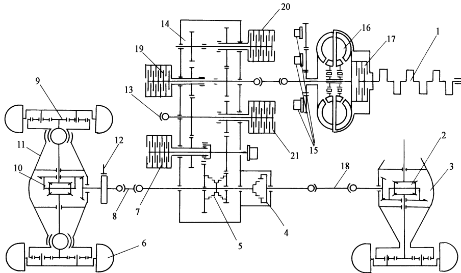
图 1 履带轮式推土机传动系
