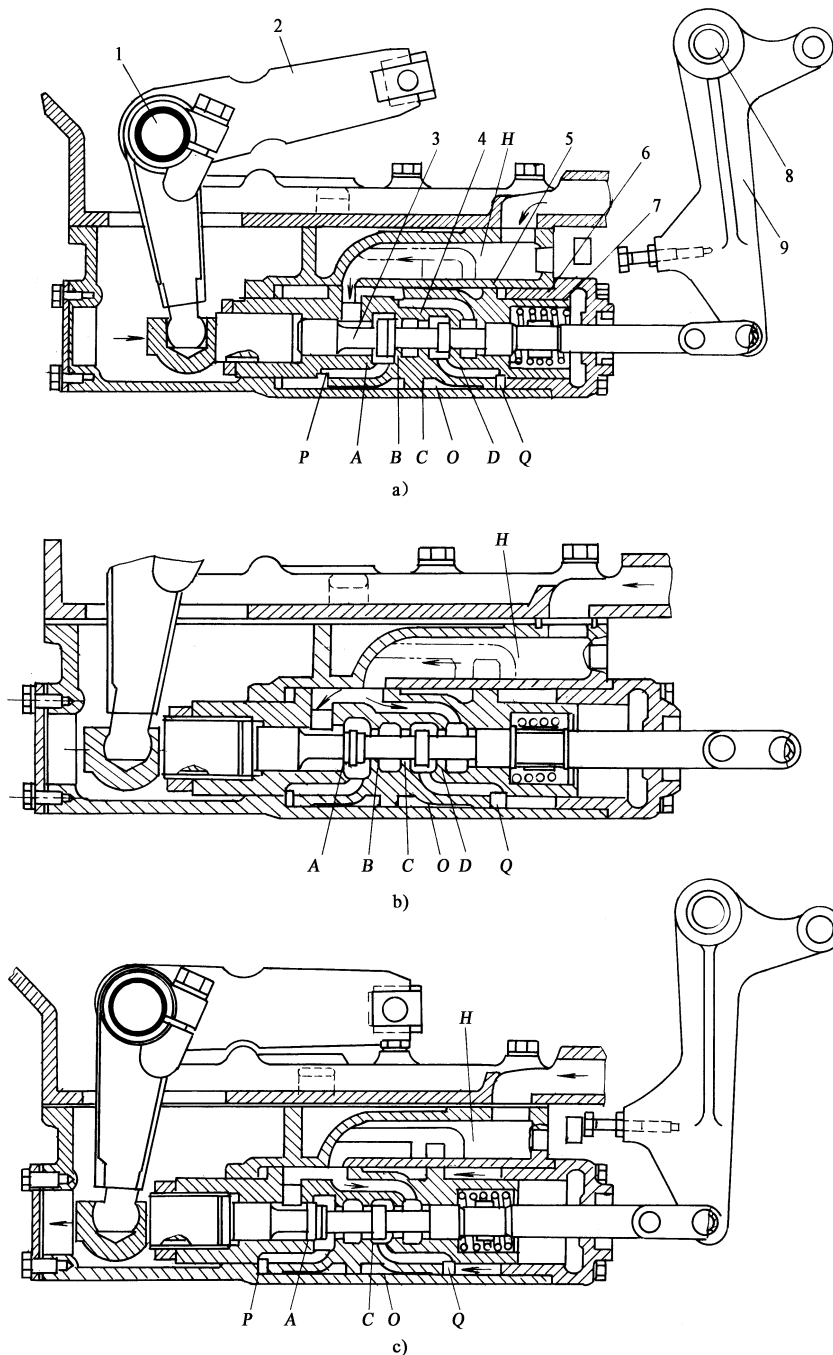
图 10-10 液力助力器
