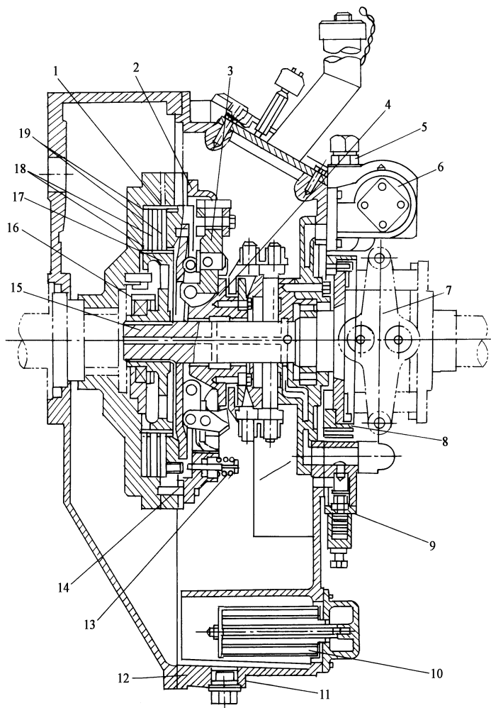
图 1-1 上海 320 型履带推土机的多片湿式主离合器
