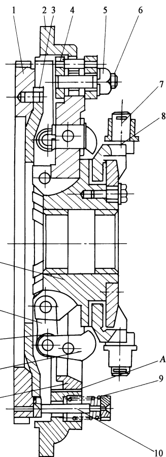
图 15-15 压紧、分离机构
