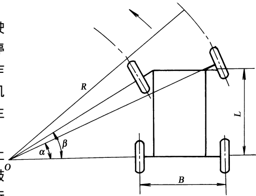
图 2 偏转车轮转向方式的示意图
