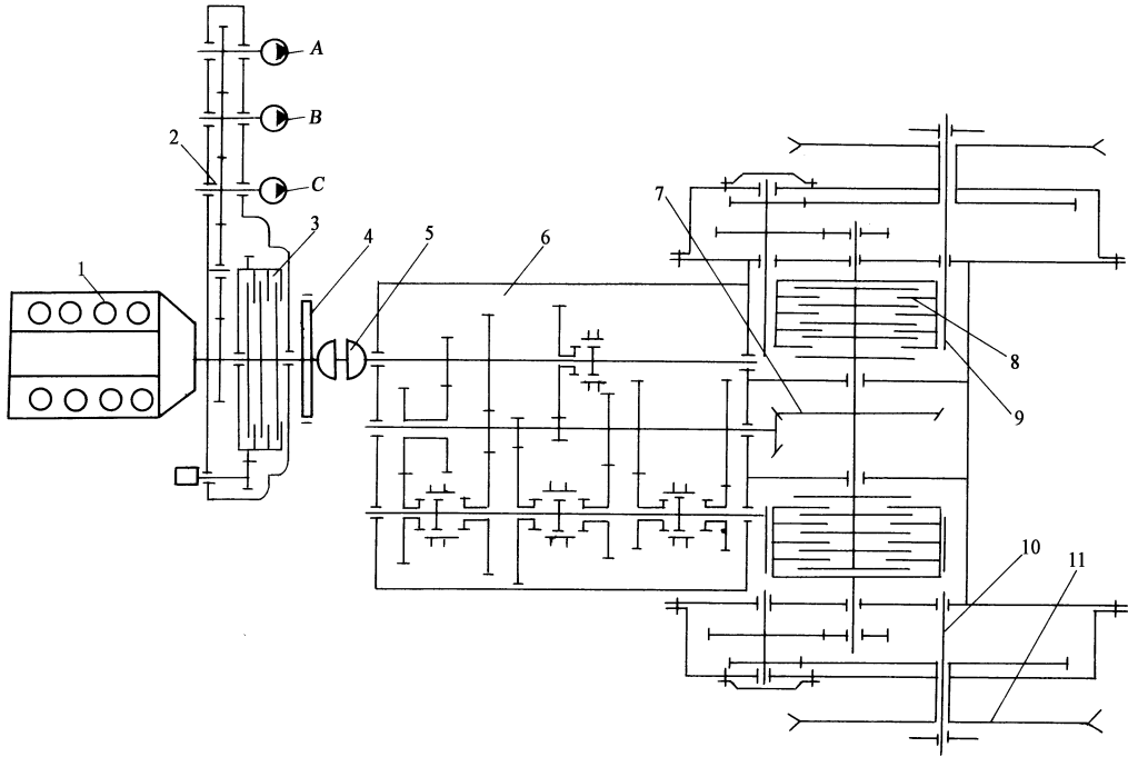
图 远 耕履带推土机传动系布置简图
