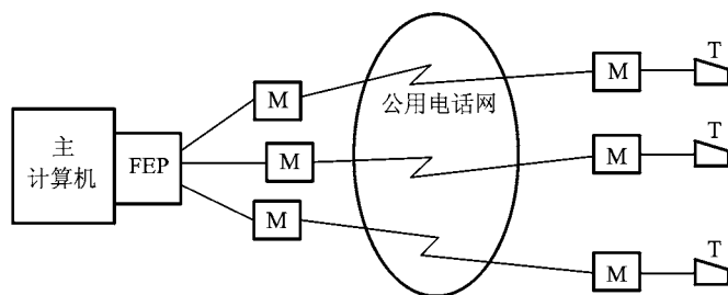
图 1-1 面向终端分布的计算机通信网
