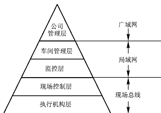
图 1-4 工业网络的体系构架
