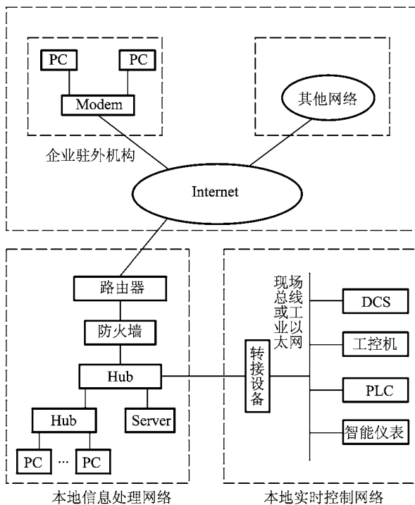
图 1-5 工业网络的一般结构
