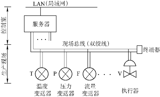
图 愿 现场总线数字仪表一对多连接
