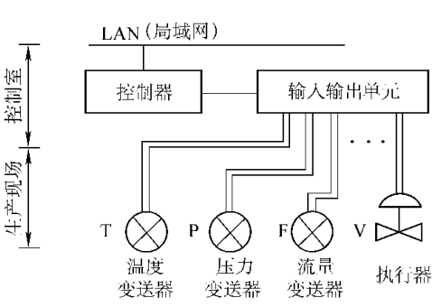
图 愿 现场常规模拟仪表一对一连接
