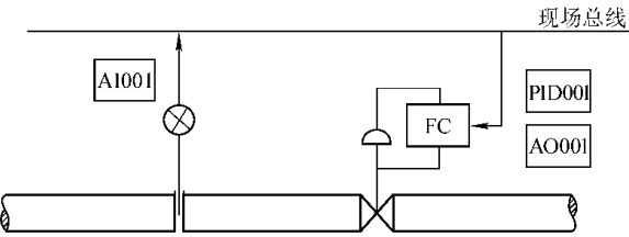
图 愿 由现场总线数字仪表实现流量控制
