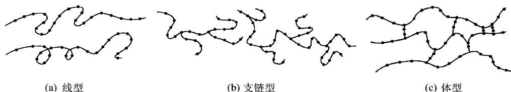
图 1 天然高分子化合物大分子的几何形状示意图
