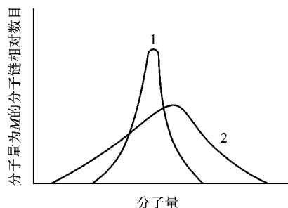
图 圆原 摇 高分子化合物的分子量分布曲线 员—分散性小 圆—分散性大
