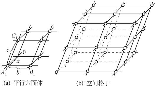
图 1-6 空间格子
