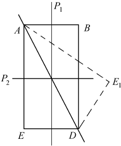
图 1-17 对称面示意
