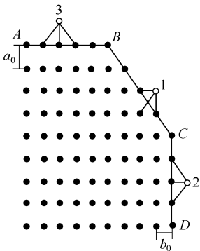
图 1-13 面网密度小的晶面优先生长的图解
