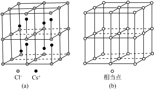
图 1-3 氯化铯的晶体结构 (a) 与空间格子 (b)
