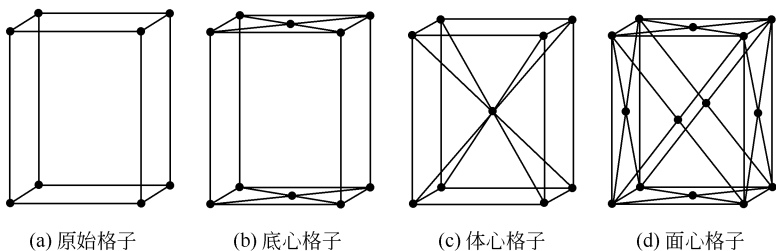
图 1-8 4 种格子类型
