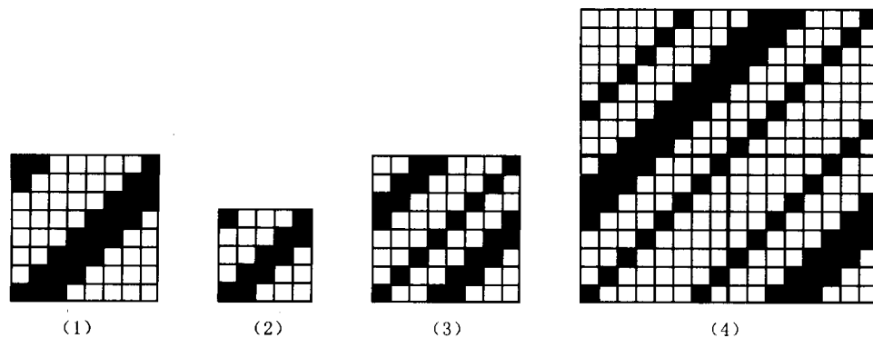
图 2-6 加强、复合斜纹
