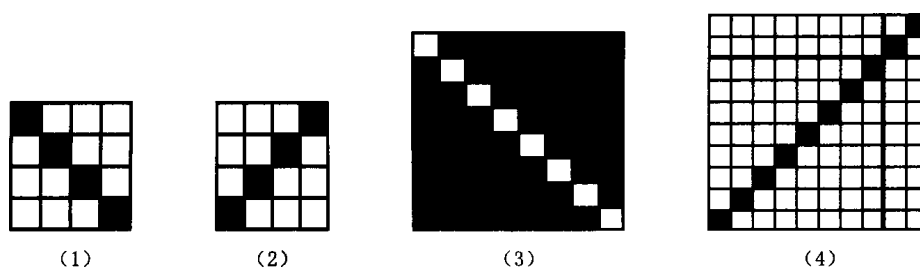
图 2-5 斜纹组织
