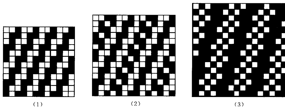
图 2-8 急斜纹及急斜纹变化组织
