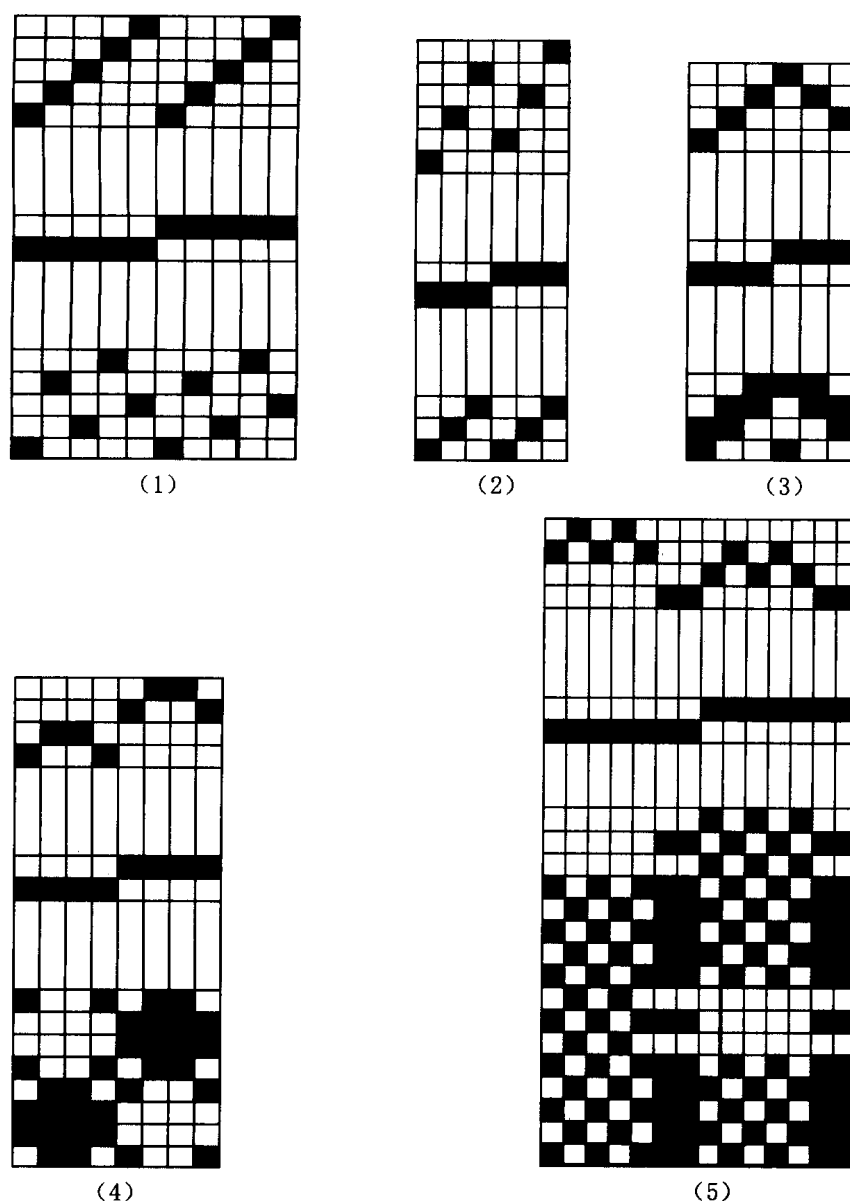
图 1-6 穿综图
