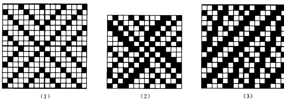
图 2-7 重叠斜纹组织
