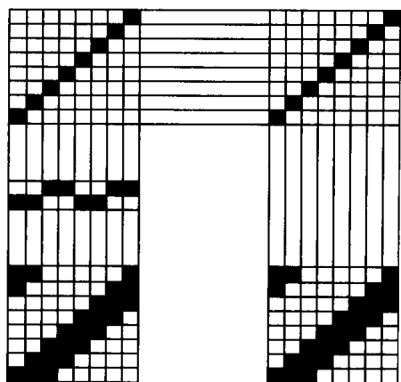
图 1-3 已知组织图、穿综图做纹板图
