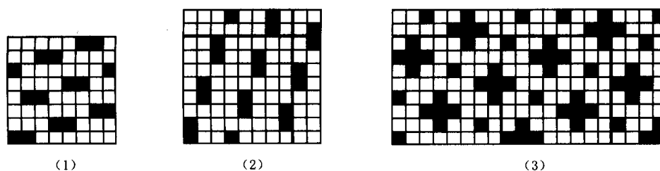
图 2 - 13 加强缎纹
