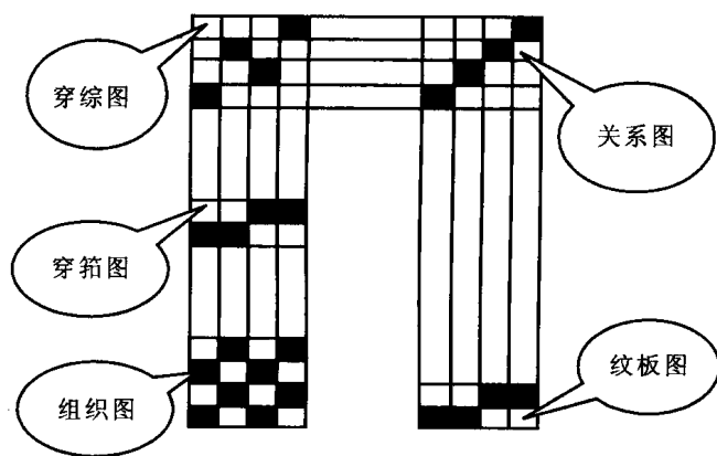
图 1-2 织物上机图
