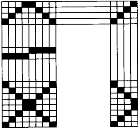
图 1-4 已知组织图、纹板图做穿综图
