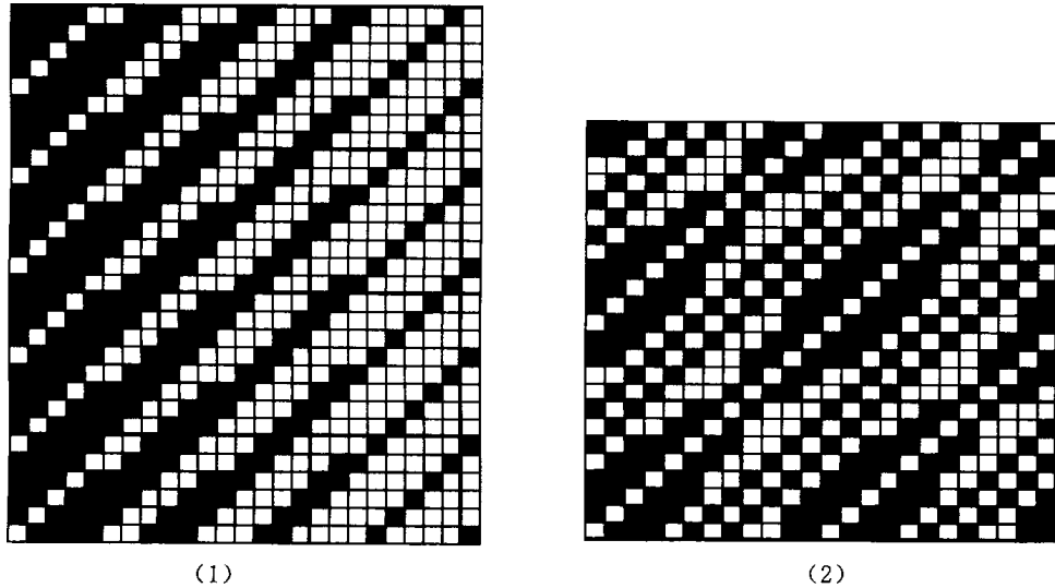
图 2 - 11 增、减经纬组织点变化斜纹
