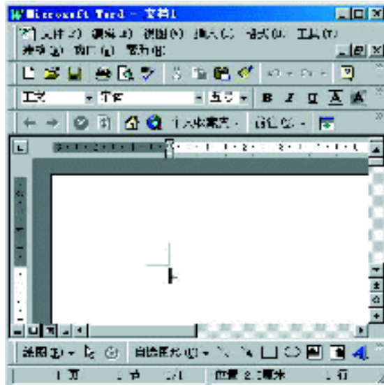
图 1-4 Word97窗口
