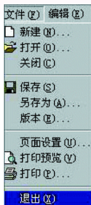
图 1-7 退出菜单
