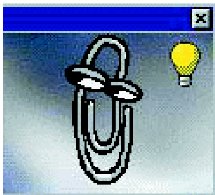
图 1-8 Office助手
