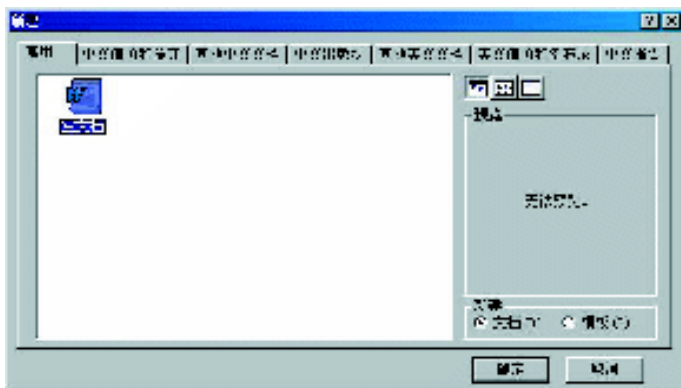
图 2-4 “新建”对话框
