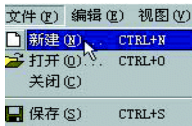
图 2-3 “新建”菜单
