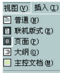
图2-5“视图”菜单
