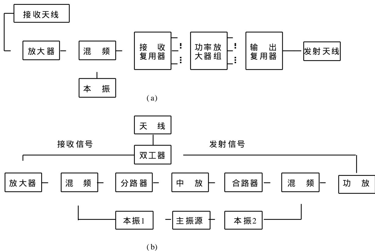
图1.6.6 透明转发器原理方框图
