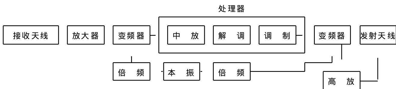
图1.6.7 处理转发器原理方框图
