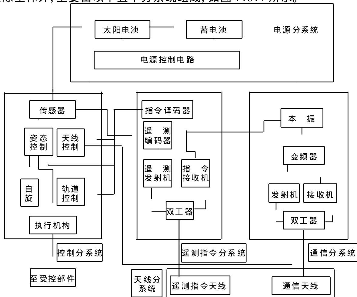
图1.6.4 通信卫星组成
