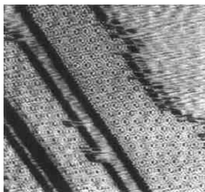
图 2-11 在 860℃ 时用 STM 实时地观察 S(111) 表面上形成 7nm×7nm 结构的重构过程
