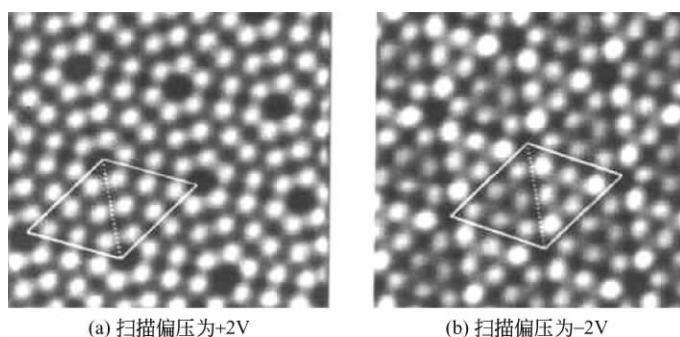
图 2-10 在超高真空的条件下，STM 得到的 Si(111)7nm×7nm(硅) 表面的原子图像
