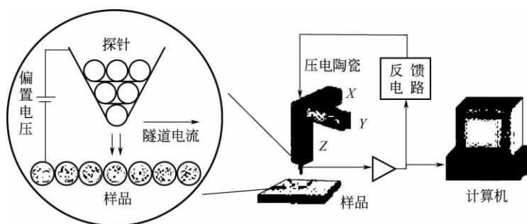
图 2-7 STM 的工作原理图
