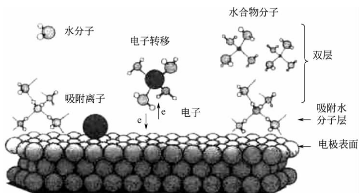
图 2-13 溶液中液/固界面上原子和分子之间发生化学反应的示意图
