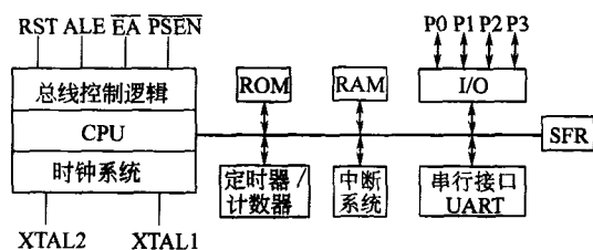
图 2-1 80C51 基核的基础结构
