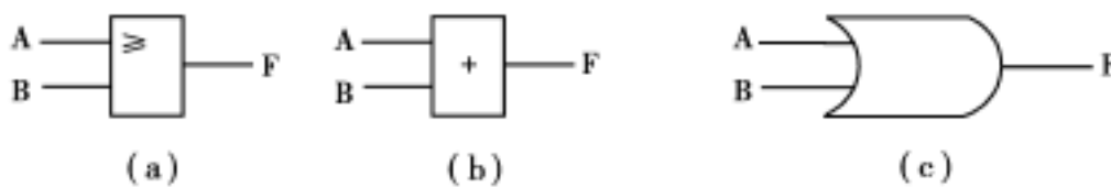
图 1.5 “或”门逻辑符号
