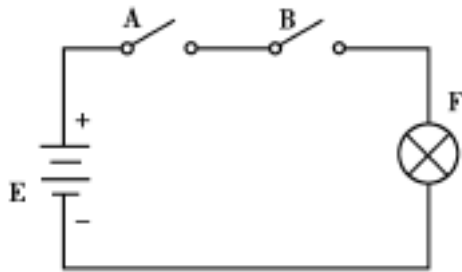
图 1.2 “与”逻辑示例
