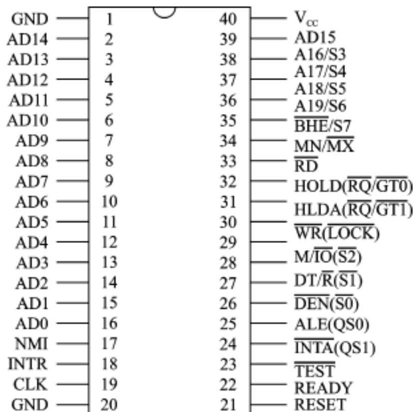
图 2.3 8086CPU 的引脚信号
