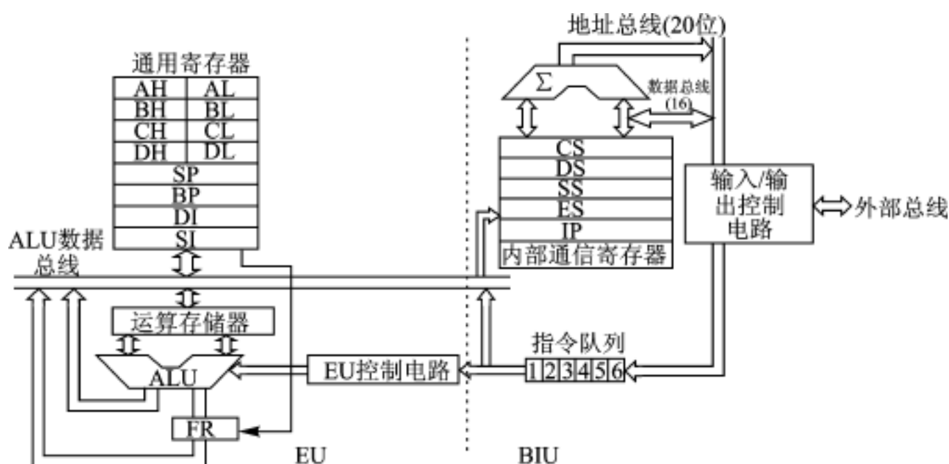
图 2.1 8086CPU 内部结构框图
