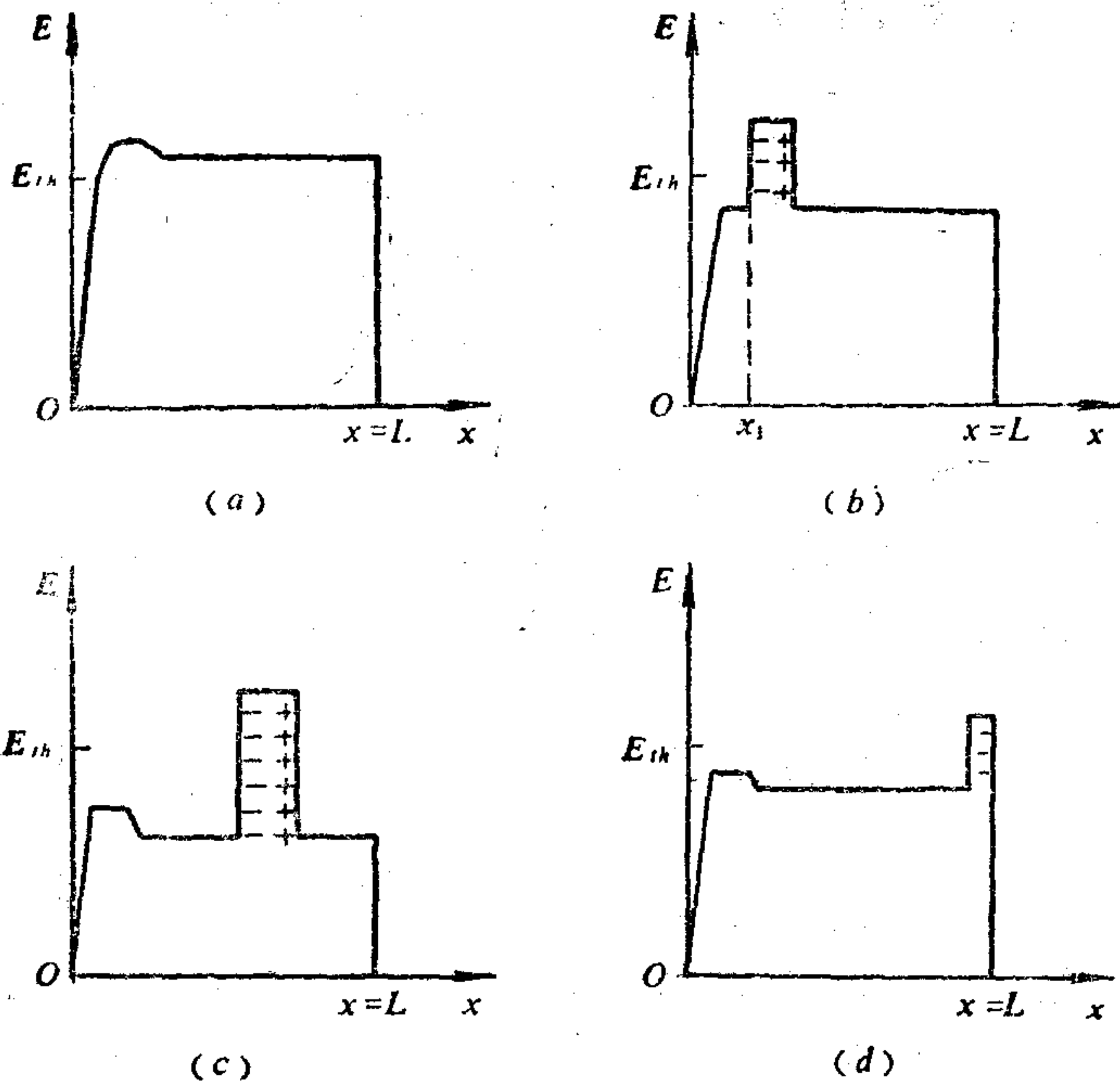
图 1-2-4 偶极畴的形成、渡越和消失过程
