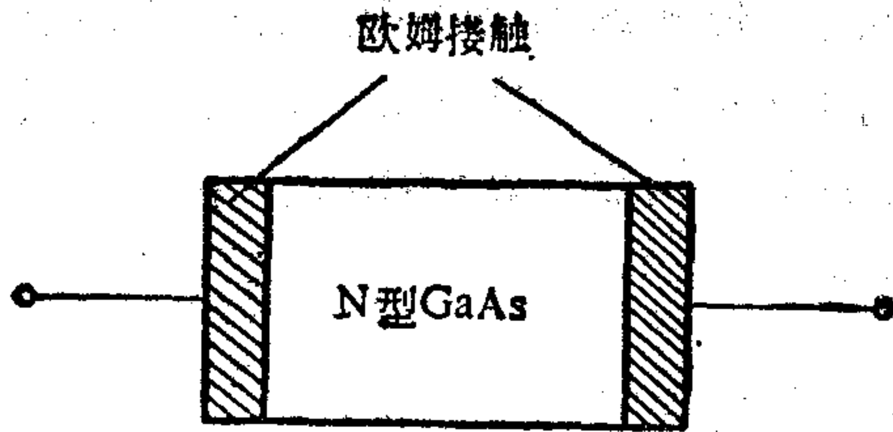
图 1-2-1 N型砷化镓转移电子器件示意图
