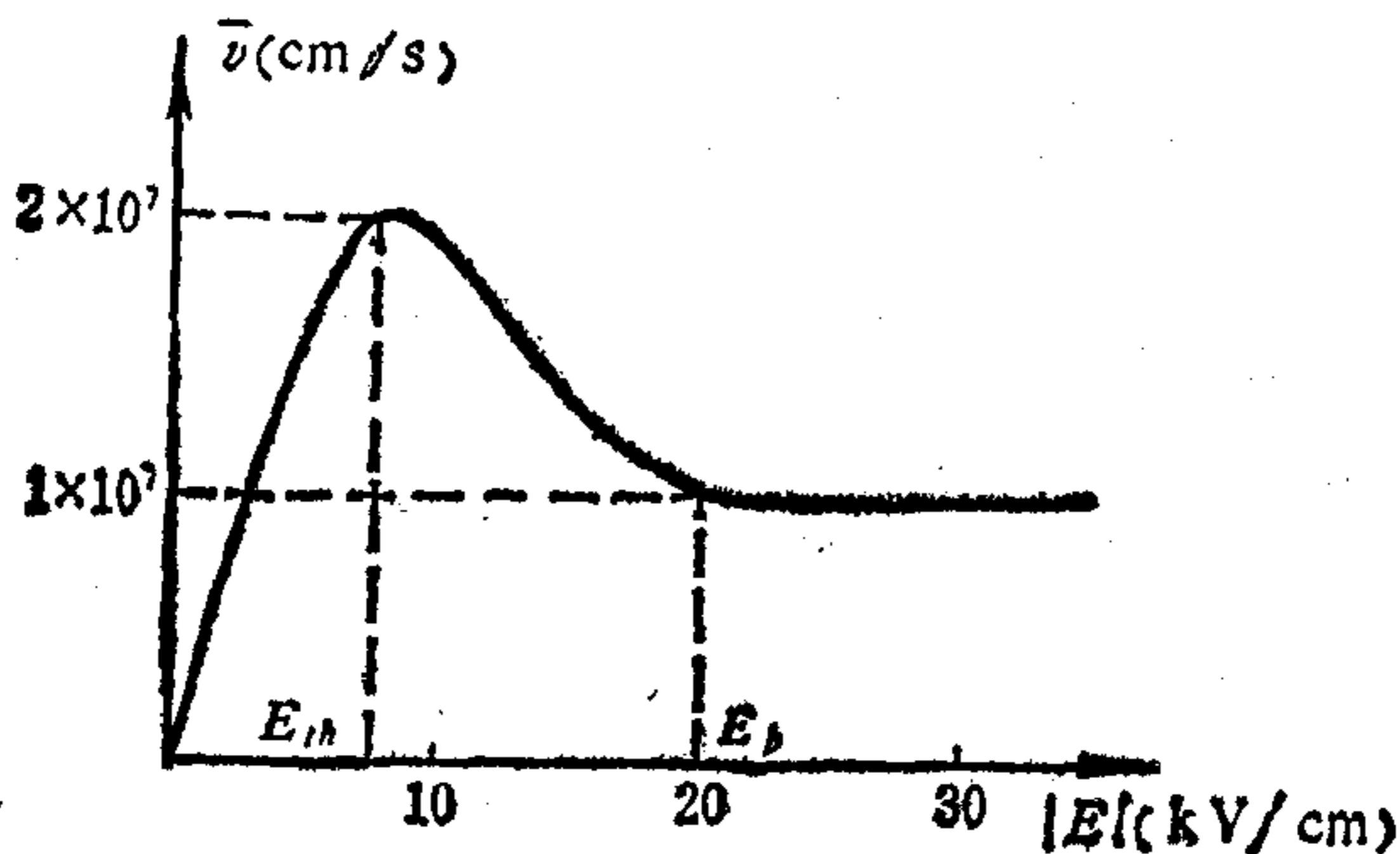
图 1-2-3 砷化镓晶体中电子的速度-电场特性
