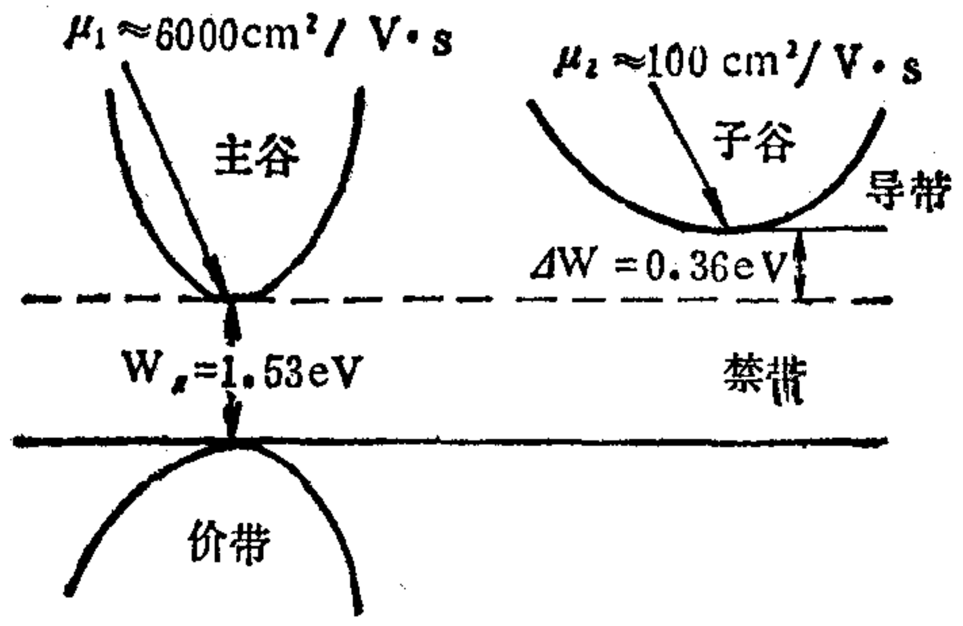
图 1-2-2 N型砷化镓的能带结构图
