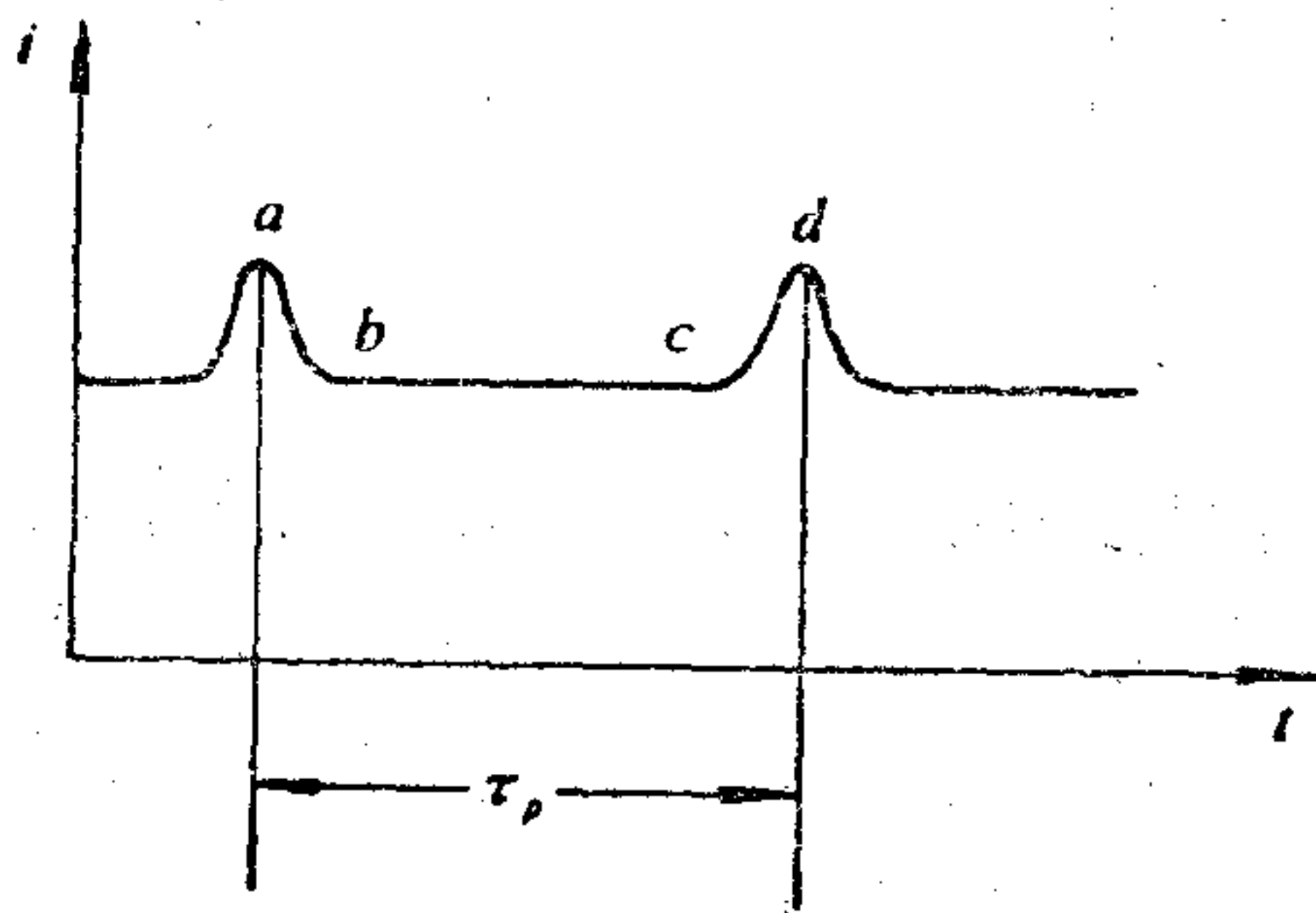
图 1-2-5 偶极畴振荡的电流波形
