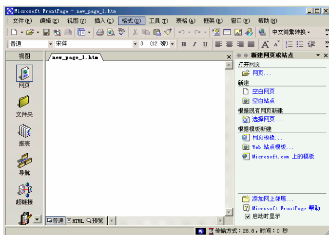
图 1-1 FrontPage 2002 窗口
