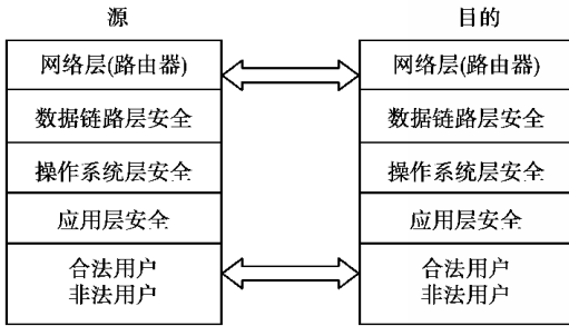
图 1-1 网络系统安全体系
