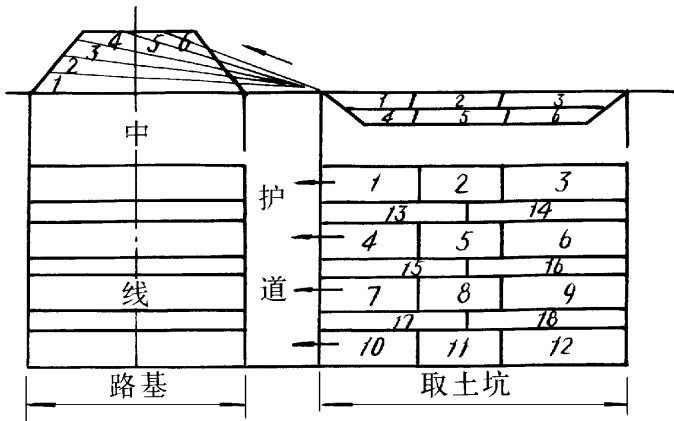
图 1—1—5 斜层填筑路堤施工程序
