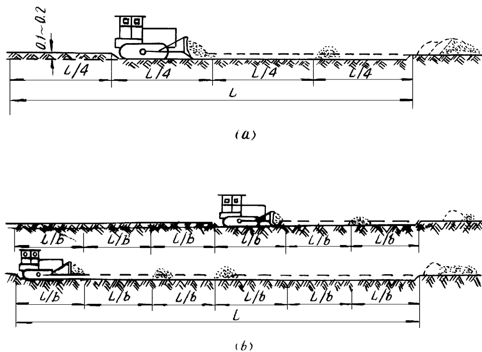
图 1—1—3 多刀推土填筑路堤 (单位: m) (a) 四刀推土; (b) 六刀推土。L——推土距离。
