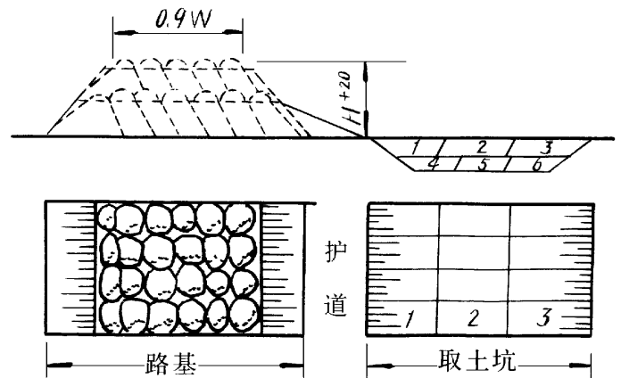
图 1—1—6 堆填法填筑路堤 (单位: m) W——路面宽度; H——路基高度。
