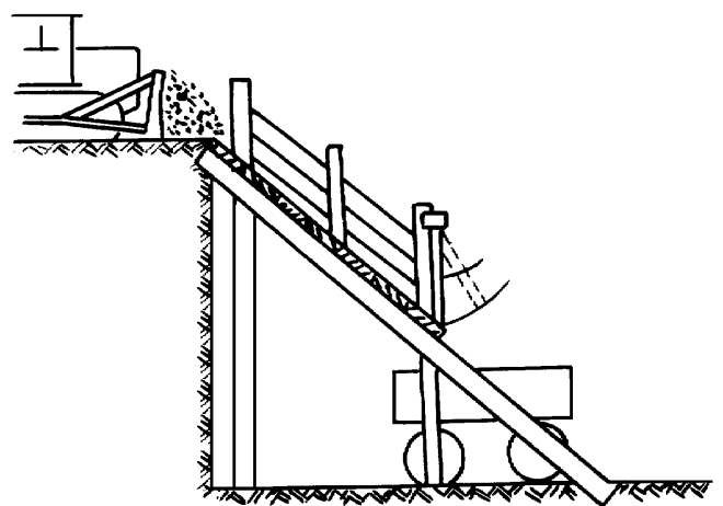
图 1—1—16 高坡滑槽装土
