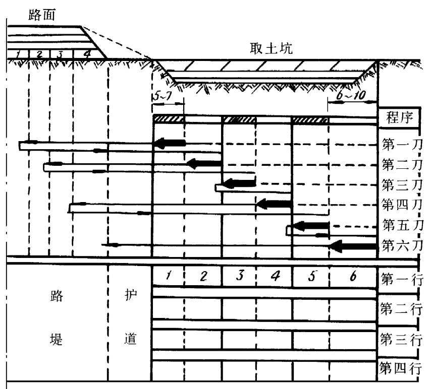
图 1—1—2 多刀推土
