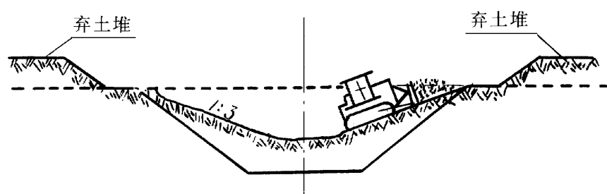
图 1—1—9 横向弃土开挖路堑
