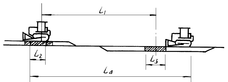
图 1—1—8 实际水平运距 L_1 ——定额水平运距; L_2 ——散土长度; L_3 ——切土长度; L_4 ——实际水平运距。
