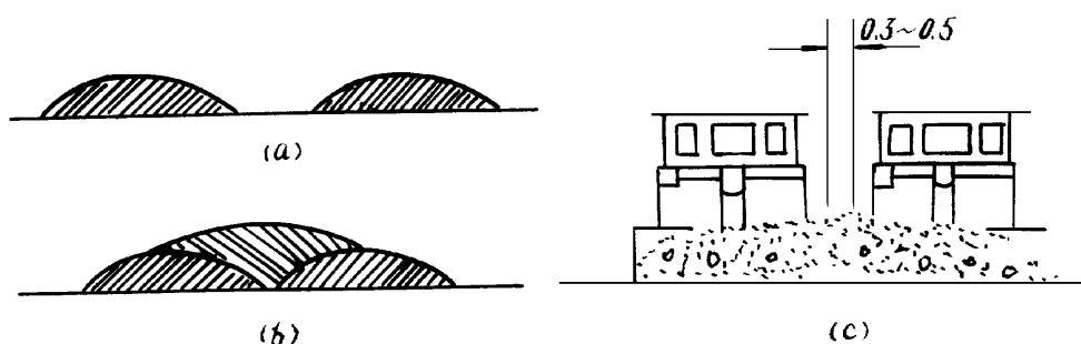
图 1—1—4 并列推土 (单位: m) (a) 单机作业推土量; (b) 并排作业推土量; (c) 双机并列作业推土量。
