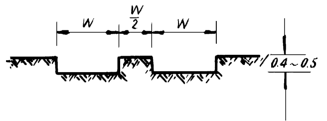
图 1—1—1 拉槽推土（单位：m）
