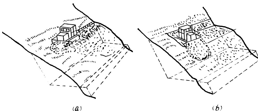
图 1—1—10 傍坡半路堑开挖
