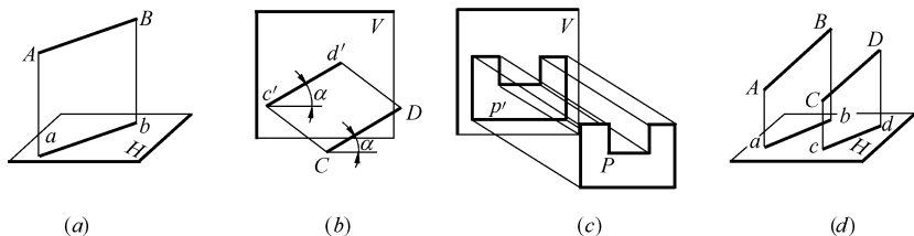
图 园缘 正投影的基本性质——不变性 (葬) 水平线；(遭) 正平线；(糟) 正平面；(凿) 两平行线
