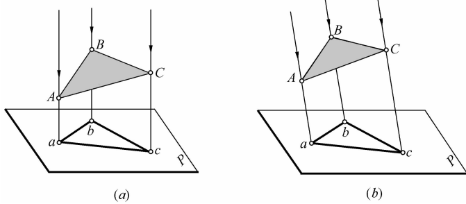
图 1-1 平行投影法
