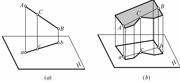
图 1-1 正投影的基本性质——从属性和定比性 (a) 直线上的点；(b) 平面上的点
