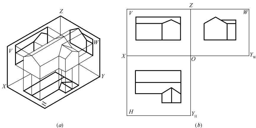
图 10-20 形体的三面投影 (a) 轴测图；(b) V 、 H 、 W 三面投影图
