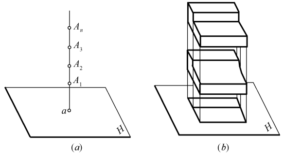
图 1-2 单面投影不能完全确定投影对象的空间位置或形状 (a) 点的单面投影；(b) 形体的单面投影
