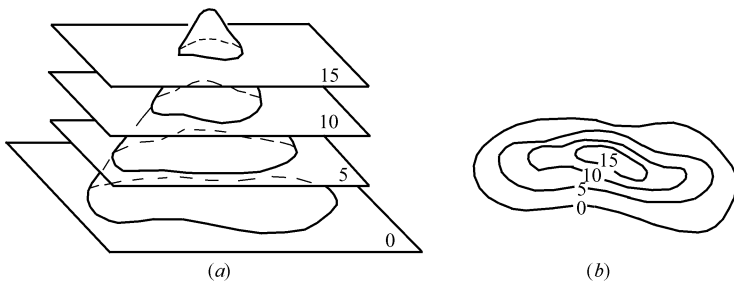
图 10-1 标高投影图
