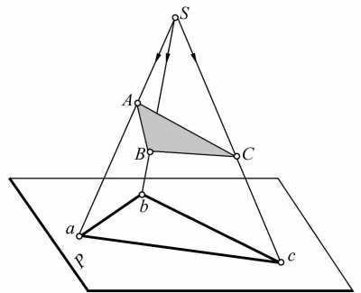
图 1-2 中心投影法
