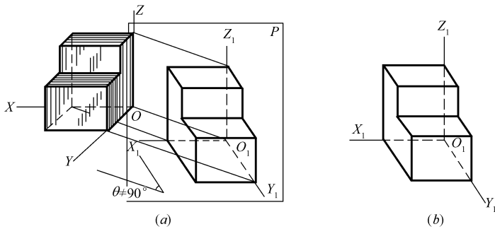
图 10-11 斜轴测图 (a) 轴测投影形成；(b) 轴测投影图
