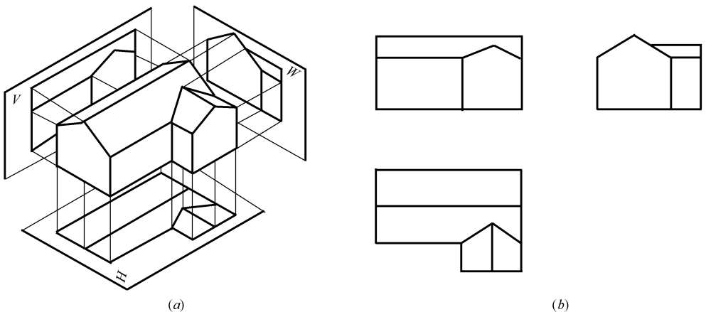
图 1-2 正投影的基本性质
