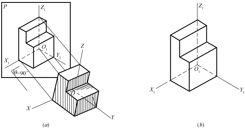
图 10-10 正轴测图 (a) 轴测投影形成；(b) 轴测投影图
