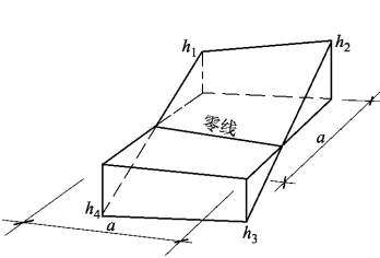
图 1-6 两挖和两填的方格
