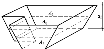
图 1-11 基坑土方量计算简图
