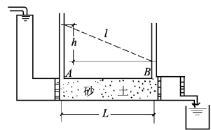
图 1-1 砂土渗透实验
