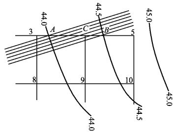
图 1-3 内插法的图解法
