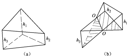
图 1-8 三角棱柱体法 (a)全挖或全填 (b)有挖有填
