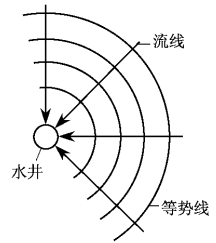
图 1-14 流网示意图
