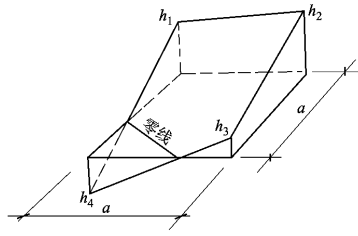
图 1-7 三挖一填(或相反)的方格
