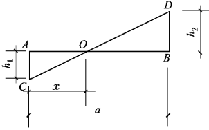
图 1-4 求零点的图解法
