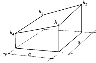
图 1-5 全挖或全填的方格
