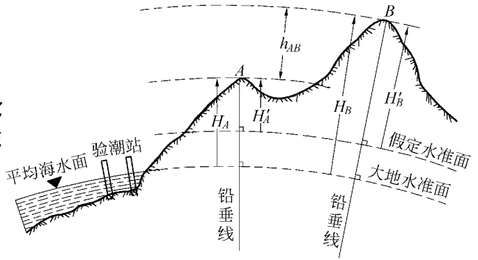
图 1-7 高程与高差的定义及其相互关系
