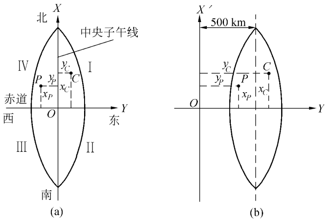
图员源 高斯平面直角坐标
