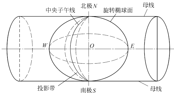
图 1-1 高斯平面直角坐标系的投影图
