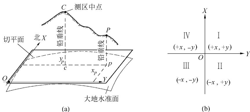
图 1-28 独立平面直角坐标系原理图
