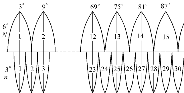
图 1-27 高斯平面直角坐标系透带投影与棱带投影的关系
