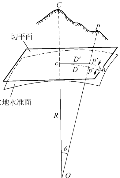
(1-9) 图 1-8 水平面代替大地水准面的影响
