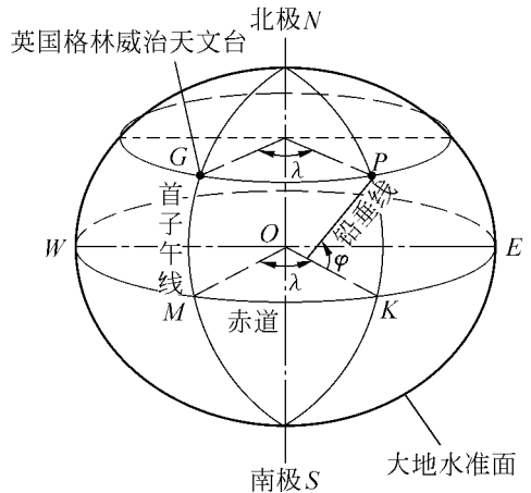
图 1-1 天文地理坐标
