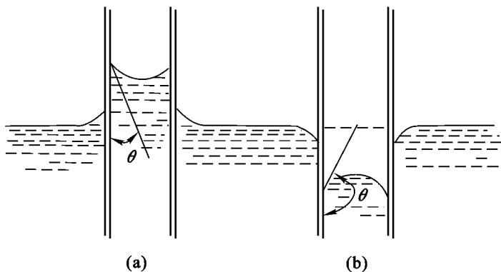
图 1-1 材料毛细管吸水性示意图
