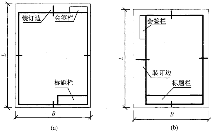
图 2 竖式图纸幅面及其尺寸代号
