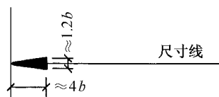
图 1-11 尺寸箭头的形式及大小
