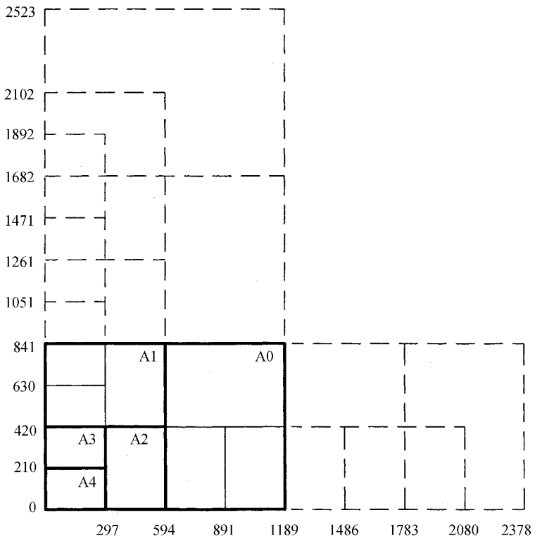
图 1 加长幅面的规定
