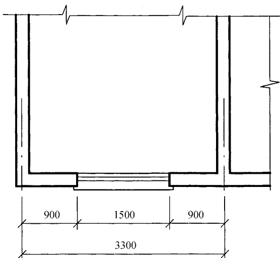
图 1-2 尺寸标注的基本形式及组成
