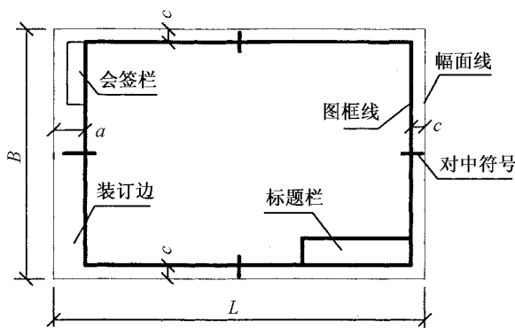
图 员圆 横式图纸幅面及其尺寸代号
