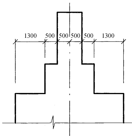
图 1-10 以轮廓线代替尺寸界线
