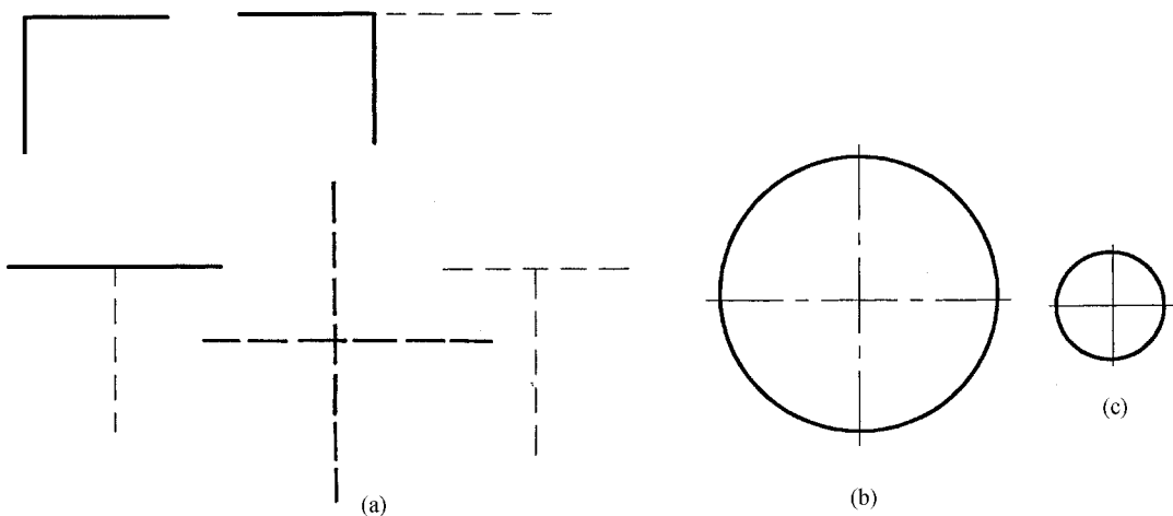
图 愿愿 实线、虚线、点画线的画法举例
