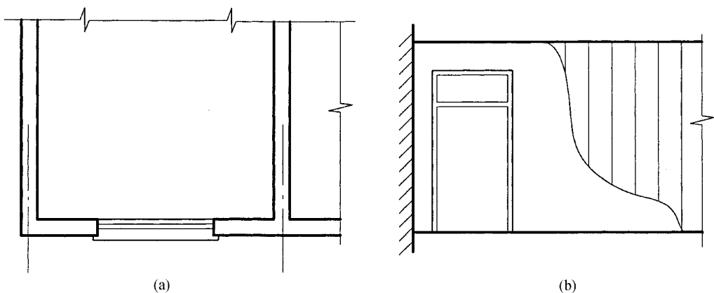
图 1-1 折断线、波浪线画法举例
