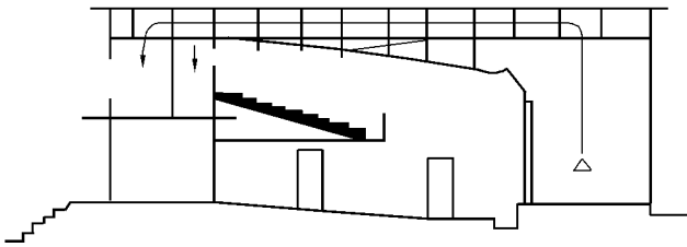
图 1-1-15 剧院内火的蔓延示意图
