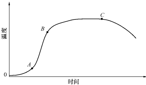
图 员原员 以时间-温度曲线表示的室内火灾发展示意图
