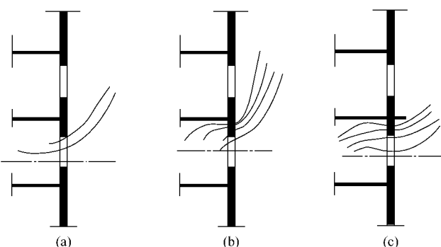
图 1-1-1 火由外墙窗口向上蔓延
