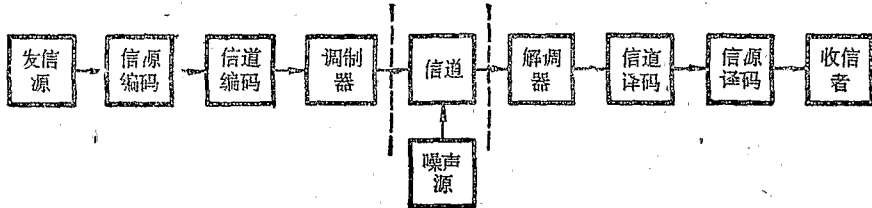
图 1-3 数字通信系统的组成
