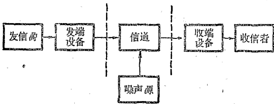
图 1-1 通信系统的组成
