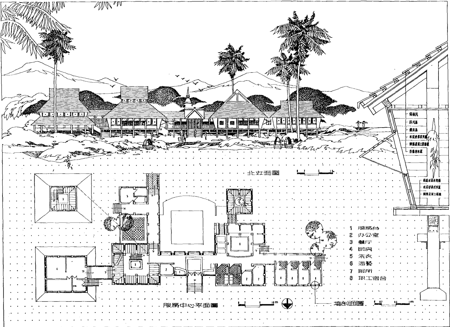
休憩客舍——云南西双版纳地区、四川峨眉山地区 台湾“洪四川”文教基金会 1990 年“优秀建筑人才奖”设计奖 1986 级本科生 郭晓东 获佳作奖 黑白钢笔墨线
