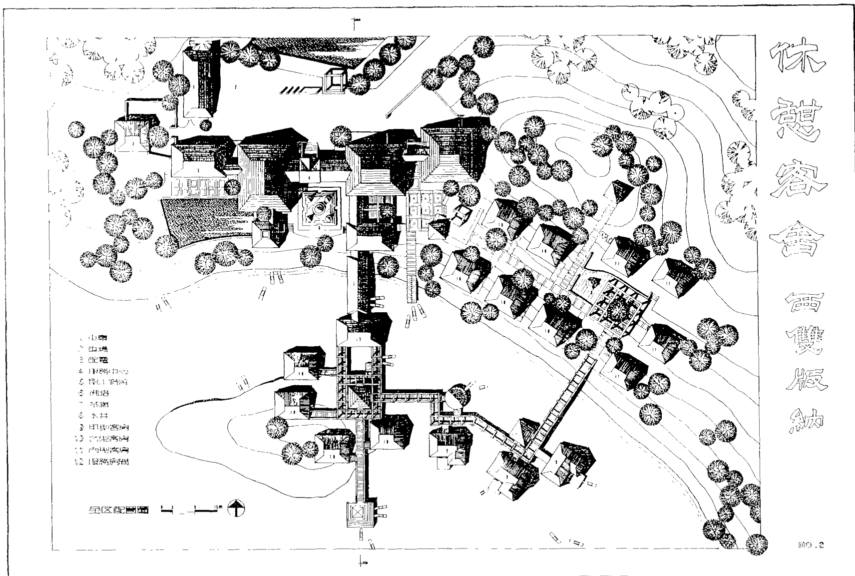
休憩客舍——云南西双版纳地区、四川峨眉山地区 台湾“洪四川”文教基金会 1990年“优秀建筑人才奖”设计奖 1986级本科生 郭晓东 获佳作奖 黑白钢笔墨线
