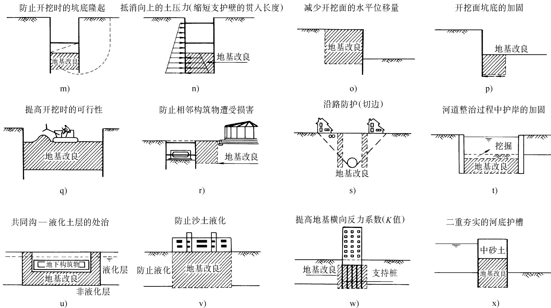
图 1-1 可供采用水泥土搅拌法加固地基的工程类型
