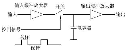
图 2-4 采样保持电路原理图
