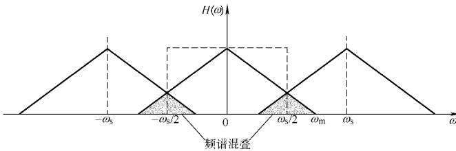
图 2-3 频谱混叠失真
