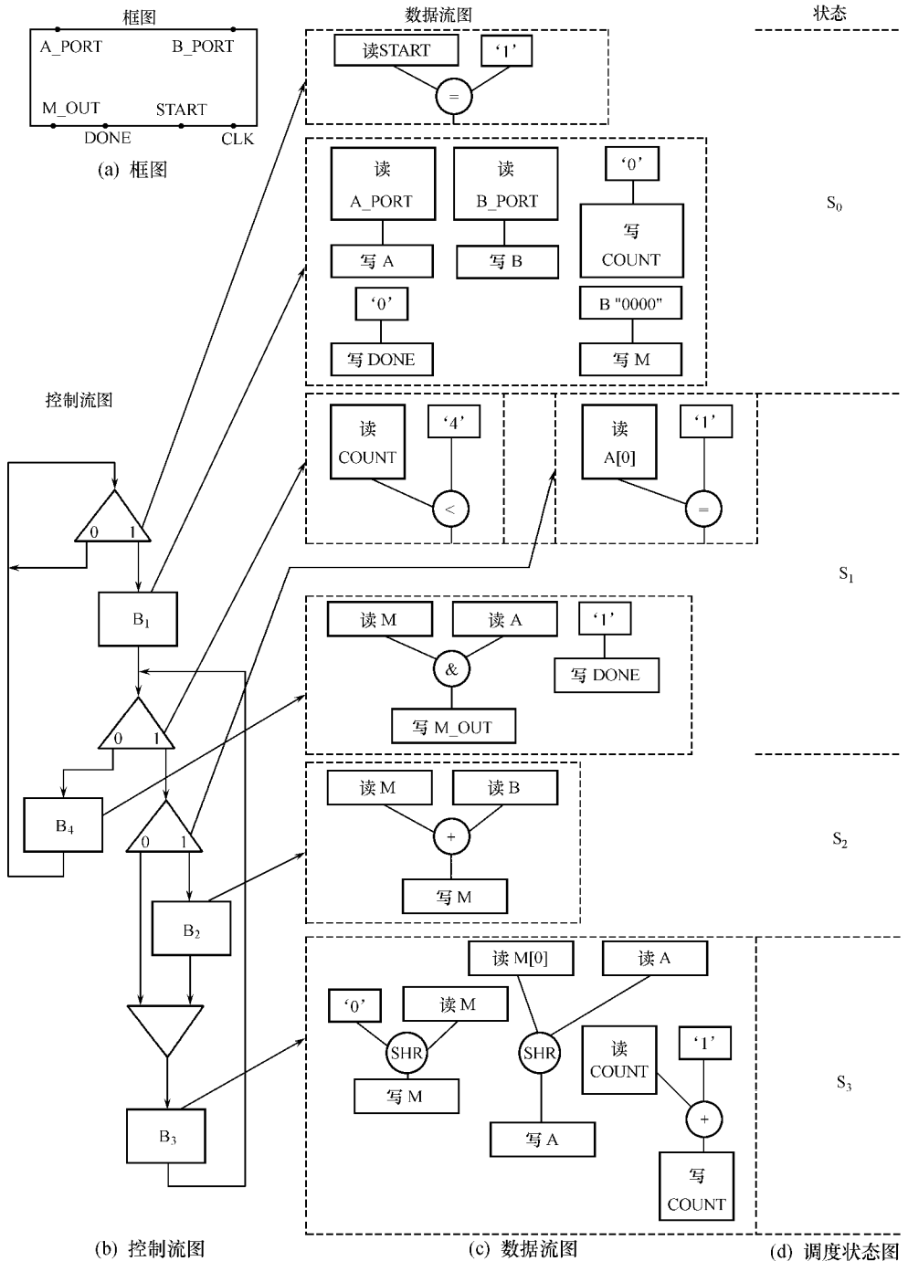
图 1-4 移位加乘器的 CDFG
