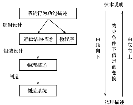
图1-1 由顶向下及由底向上设计过程
