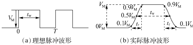
图 1.1 脉冲波形
