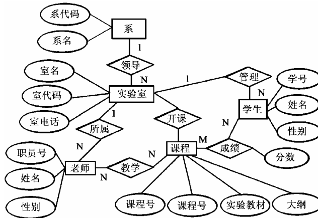
图 1-4 学校实验室教学系统的 E-R 图
