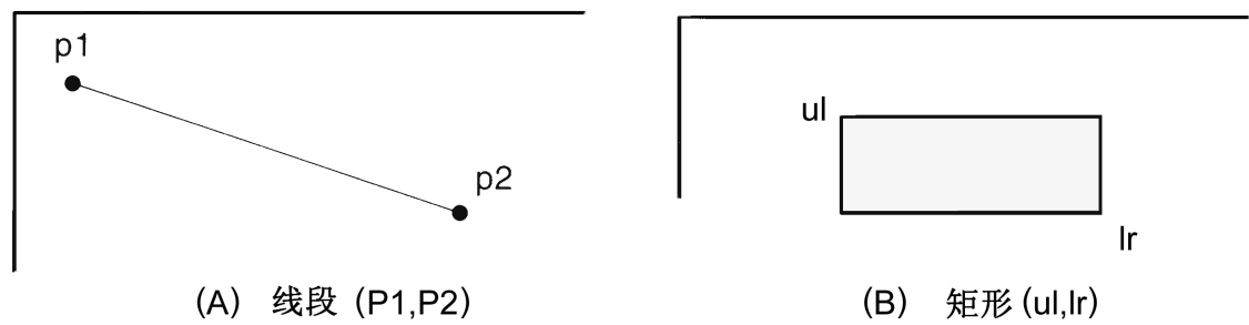
图 1.1 线段和矩形
