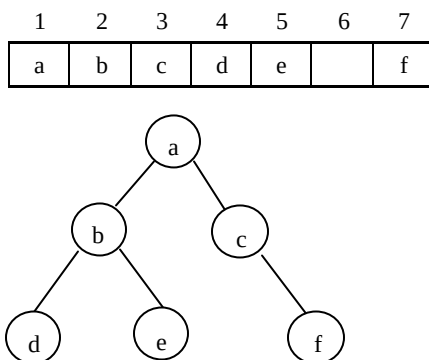
图 1.1 一颗二叉树
