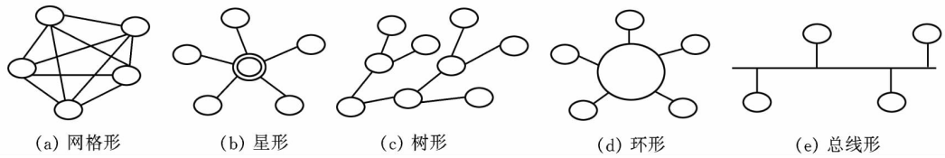
图 1.9 数据通信网的几种典型拓扑结构
