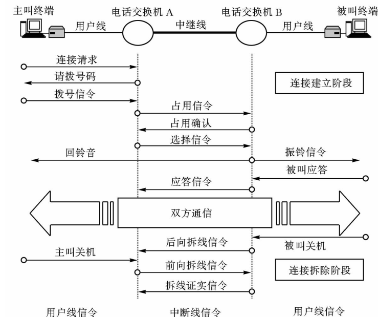
图 1.7 利用电话网进行一次数据通信过程
