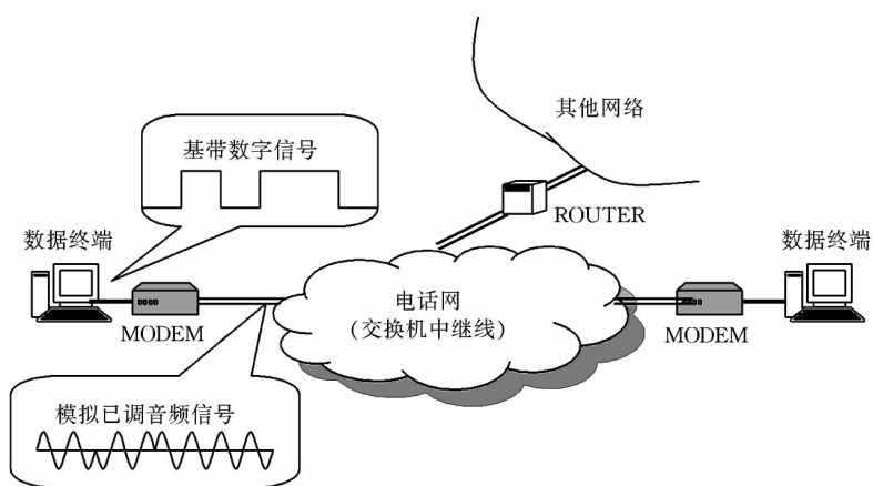
图 1.6 利用电话网进行数据通信
