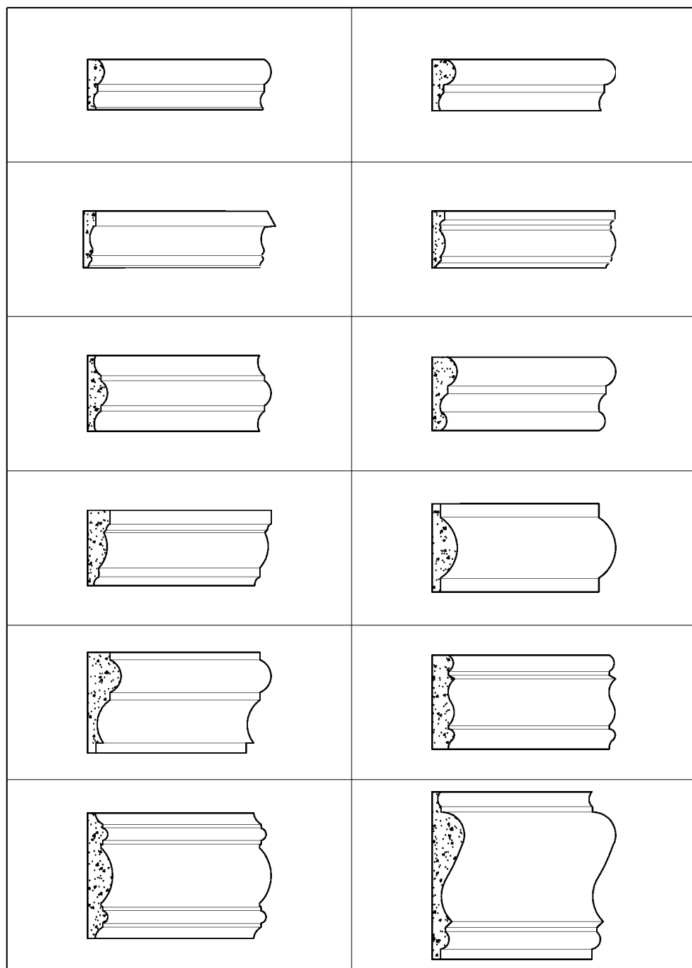
图 8-1 天然石材饰线
