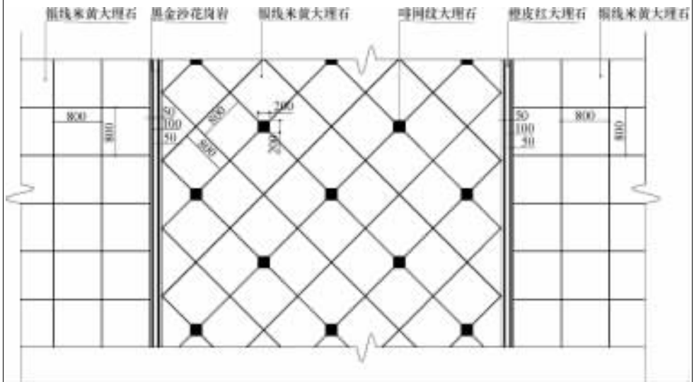
图 圆藏器地面石材拼花
