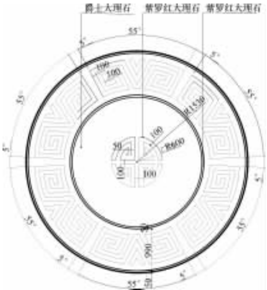
图 圆藏器地面石材拼花
