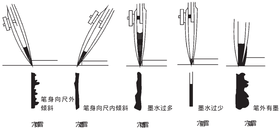
图 员原猿 直 线笔使用不当 的几种情况
