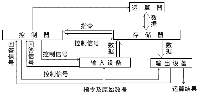
图员圆缘圆计算机基本结构示意图
