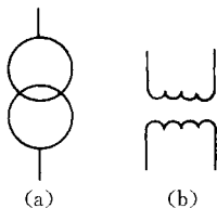
图 1-3 变压器 (a) 单线形式； (b) 多线形式
