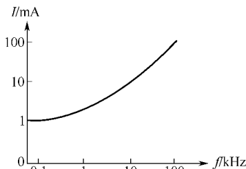
图 1.4 电流刺激的阈值与频率的关系
