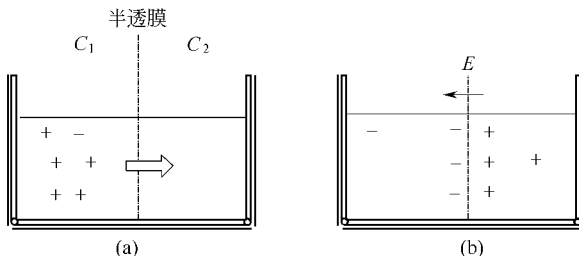
图 2.2 扩散形成的能斯特（Nernst）电动势
