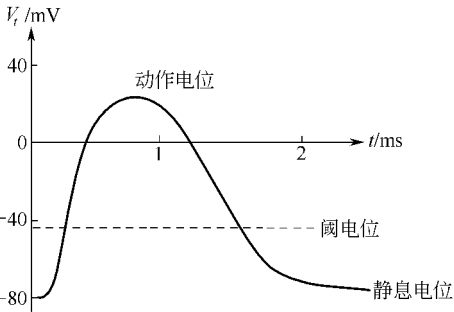
图 2.1 无脊椎动物轴突动作电位
