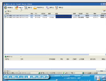
➤ 电驴软件
