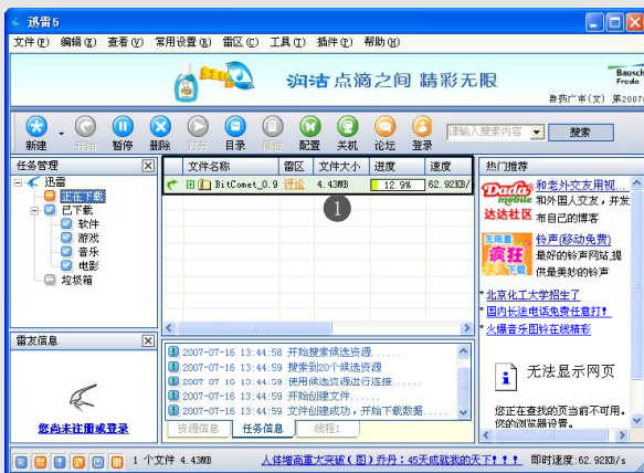
图 4-5 开始下载
